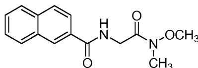
N -(2-(methoxy(methyl)amino)-2-oxoethyl)-2-naphthamide
