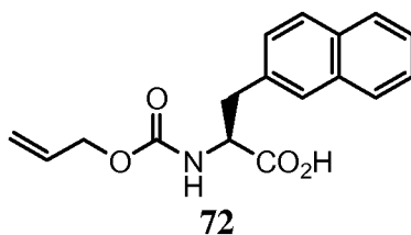
((S)-2-(allyloxycarbonylamino)-3-(naphthalen-2-yl)propanoic acid
