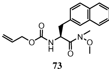
(S)-allyl 1-(methoxy(methyl)amino)-3-(naphthalen-2-yl)-1-oxopropan-2-ylcarbamate
