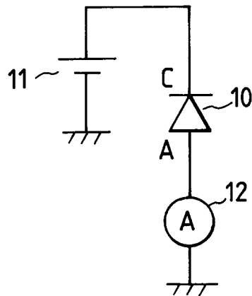
FIG. 16C
