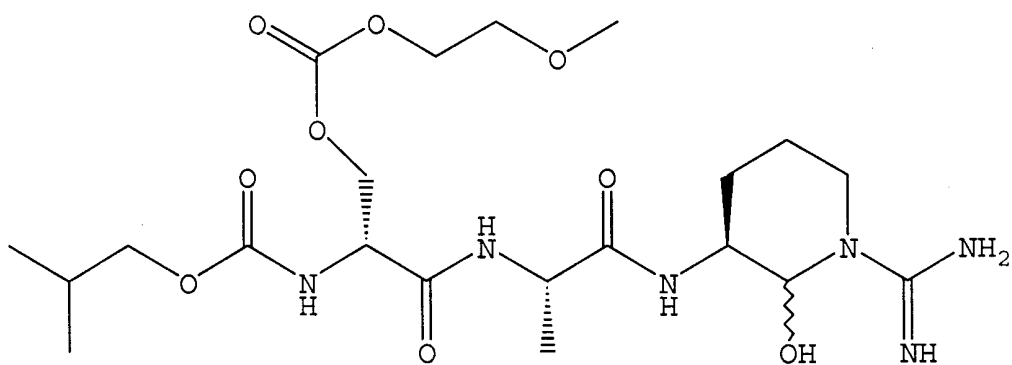
isobutoxycarbonyl-D- (2-methoxyethoxycarbonyl) -Ser-L-Ala-argininal;
