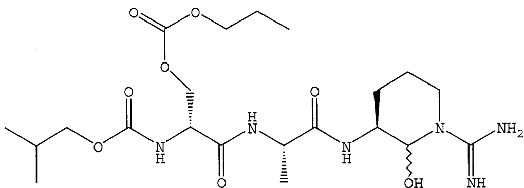
isobutoxycarbonyl-D- (n-propyloxycarbonyl) -Ser-L-Ala-argininal;
