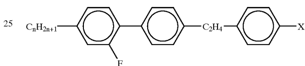
FET-nX
