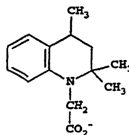
Cpd. 47
