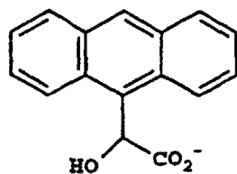
Cpd. 56
