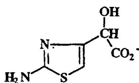
Cpd. 60
