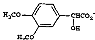
Cpd. 51
