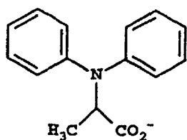
Cpd. 58
