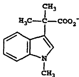
Cpd. 44
