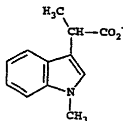
Cpd. 45
