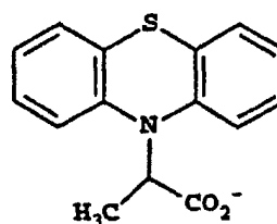
Cpd. 57
