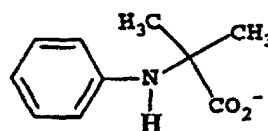
Cpd. 59
