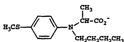
Cpd. 61
