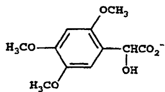
Cpd. 48
