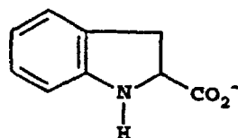
Cpd. 55
