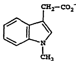
Cpd. 46
