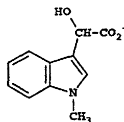
Cpd. 43
