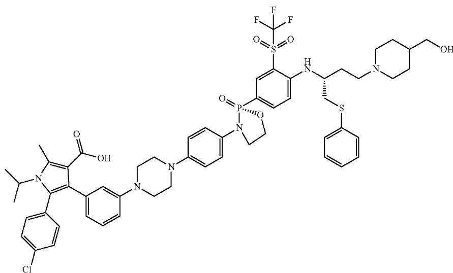
5-(4-chlorophenyl)-4-(3-(4-(4-((R)-2-(4-((R)-4-(4-hydroxymethyl)piperidin-1-yl)-1-(phenylthio)butan-2-yl)amino)-3-(trifluoromethyl)sulfonyl)phenyl)-2-oxido-1,3,2-oxazaphospholidin-3-yl)phenyl)piperazin-1-yl)phenyl)-1-isopropyl-2-methyl-1H-pyrrole-3-carboxylic acid
