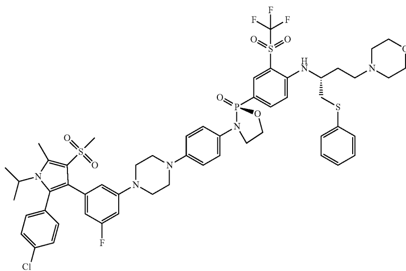
(S)-3-(4-(4-(3-(2-(4-chlorophenyl)-1-isopropyl-5-methyl-4-(methylsulfonyl)-1H-pyrrol-3-yl)-5-fluorophenyl)piperazin-1-yl)phenyl)-2-(4(((R)-4-morpholino-1-(phenylthio)butan-2-yl)amino)-3-(trifluoromethyl)sulfonyl)phenyl)-1,3,2-oxazaphospholidine 2-oxide
