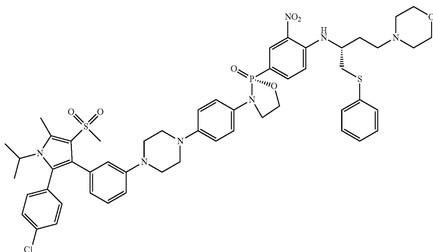
(R)-3-(4-(4-(3-(2-(4-chlorophenyl)-1-isopropyl-5-methyl-4-(methylsulfonyl)-1H-pyrrol-3-yl)phenyl)piperazin-1-yl)phenyl)-2-(4-(((R)-4-morpholino-1-(phenylthio)butan-2-yl)amino)-3-nitrophenyl)-1,3,2-oxazaphospholidine 2-oxide
