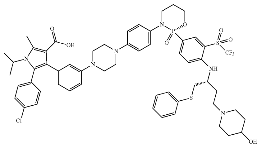
5-(4-chlorophenyl)-4-(3-(4-(4-((S)-2-4-((R)-4-(4-hydroxypiperidin-1-yl)-1-(phenylthio)butan-2-yl)amino)-3-((trifluoromethyl)sulfonyl)phenyl)-2-oxido-1,3,2-oxazaphosphinan-3-yl)phenyl)piperazin-1-yl)phenyl)-1-isopropyl-2-methyl-1H-pyrrole-3-carboxylic acid
