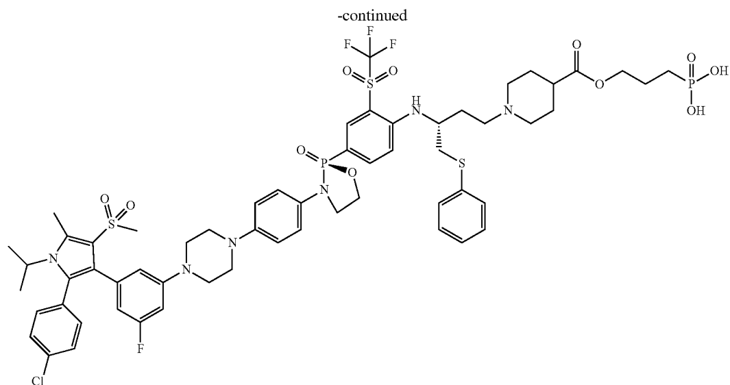
(3-((1-((R)-3-((4-((S)-3-(4-(4-(3-(2-(4-chlorophenyl)-1-isopropyl-5-methyl-4-(methylsulfonyl)-1H-pyrrol-3-yl)-5-fluorophenyl)piperazin-1-yl)phenyl)-2-oxido-1,3,2-oxazaphospholidin-2-yl)-2-((trifluoromethyl)sulfonyl)phenyl)amino)-4-(phenylthio)butyl)piperidine-4-carbonyloxy)propyl)phosphonic acid
