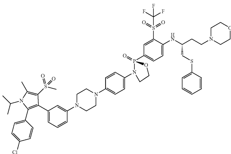
(S)-3-(4-(4-(3-(2-(4-chlorophenyl)-1-isopropyl-5-methyl-4-(methylsulfonyl)-1H-pyrrol-3-yl)phenyl)piperazin-1-yl)phenyl)-2-(4-(((R)-4-(dimethylamino)-1-(phenylthio)butan-2-yl)amino)-3-(trifluoromethyl)sulfonyl)phenyl)-1,3,2-oxazaphospholidine 2-oxide
