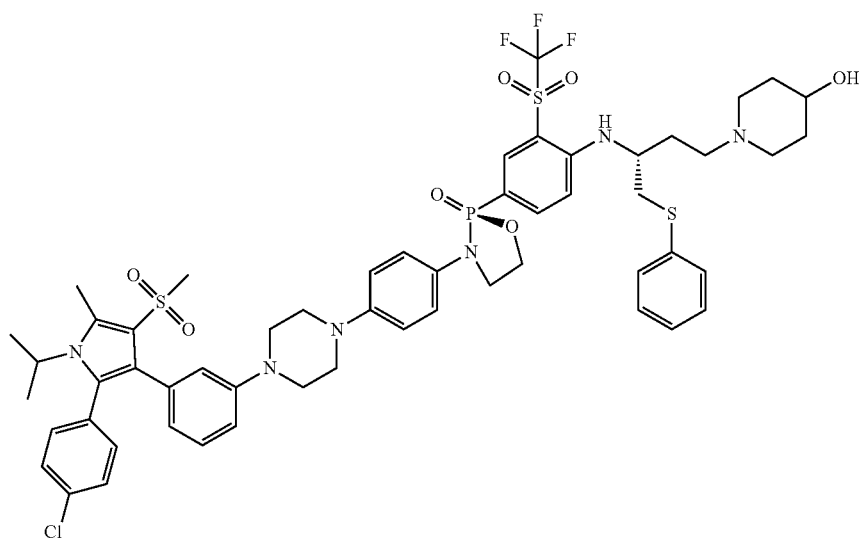
(S)-3-(4-(4-(3-(2-(4-chlorophenyl)-1-isopropyl-5-methyl-4-(methylsulfonyl)-1H-pyrrol-3-yl)phenyl)piperazin-1-yl)phenyl)-2-(4-(((R)-4-(4-hydroxypiperidin-1-yl)-1-(phenylthio)butan-2-yl)amino)-3-(trifluoromethyl)sulfonyl)phenyl)-1,3,2-oxazaphospholidine 2-oxide
