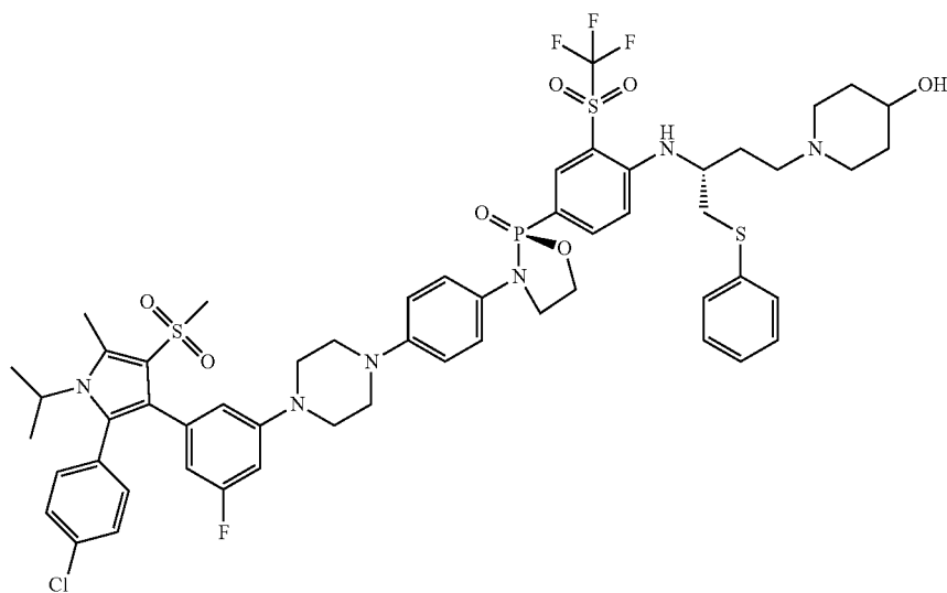
(S)-3-(4-(3-(2-(4-chlorophenyl)-1-isopropyl-5-methyl-4-(methylsulfonyl)-1H-pyrrol-3-yl)-5-fluorophenyl)piperazin-1-yl)phenyl)-2-(4-(((R)-4-(4-(hydroxypiperidin-1-yl)-1-(phenylthio)butan-2-yl)amino)-3-(trifluoromethyl)sulfonyl)phenyl)-1,3,2-oxazaphospholidine 2-oxide
