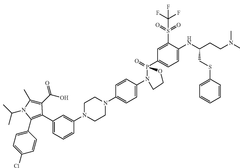
5-(4-chlorophenyl)-4-(3-(4-(4-((S)-2-4-(((R)-4-(dimethylamino)-1-(phenylthio)butan-2-yl)amino)-3-(trifluoromethyl)sulfonyl)phenyl)-2-oxido-1,3,2-oxazaphospholidin-3-yl)phenyl)piperazin-1-yl)phenyl)-1-isopropyl-2-methyl-1H-pyrrole-3-carboxylic acid
