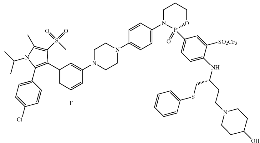
(R)-3-(4-(4-(3-(2-(4-chlorophenyl)-1-isopropyl-5-methyl-4-(methylsulfonyl)-1H-pyrrol-3-yl)-5-fluorophenyl)piperazin-1-yl)phenyl)-2-(4-(((R)-4-(dimethylamino)-1-(phenylthio)butan-2-yl)amino)-3-((trifluoromethyl)sulfonyl)phenyl)-1,3,2-oxazaphosphinane 2-oxide
