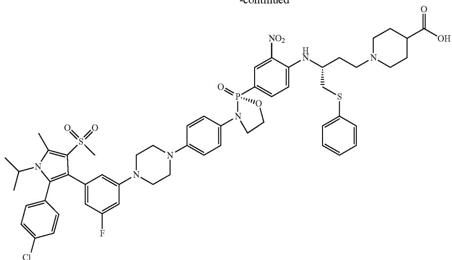
1-((R)-3-((4-((R)-3-(4-(4-(3-(2-(4-chlorophenyl)-1-isopropyl-5-methyl-4-(methylsulfonyl)-1H-pyrrol-3-yl)-5-fluorophenyl)piperazin-1-yl)phenyl)-2-oxido-1,3,2-oxazaphospholidin-2-yl)-2-nitrophenyl)amino)-4-(phenylthio)butyl)piperidine-4-carboxylic acid
