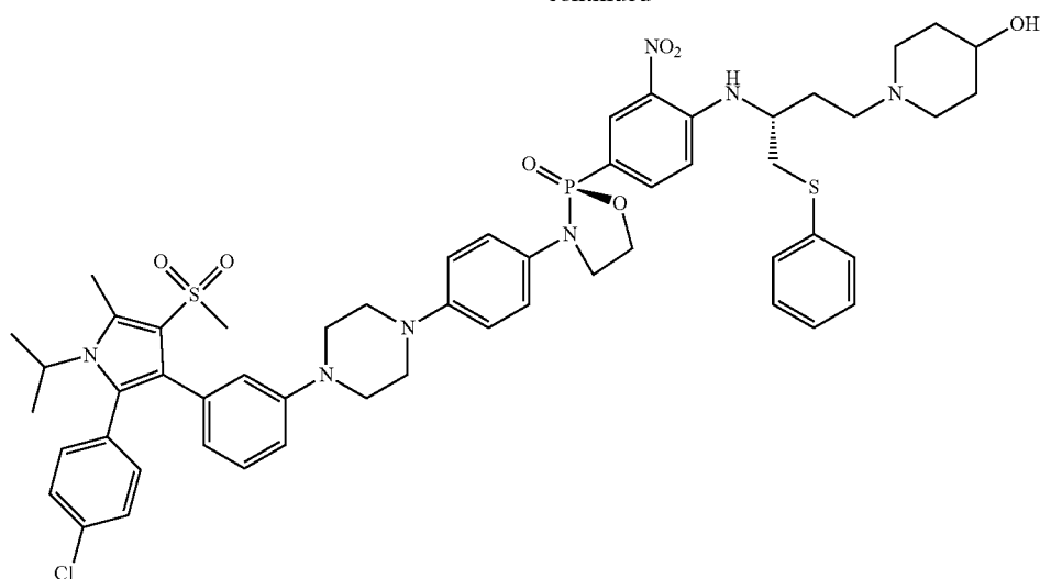
(S)-3-(4-(3-(2-(4-chlorophenyl)-1-isopropyl-5-methyl-4-(methylsulfonyl)-1H-pyrrol-3-yl)-phenyl)piperazin-1-yl)phenyl)-2-(4-(((R)-4-(4-hydroxypiperidin-1-yl)-1-(phenylthio)butan-2-yl)amino)-3-nitrophenyl)-1,3,2-oxazaphospholidine 2-oxide
