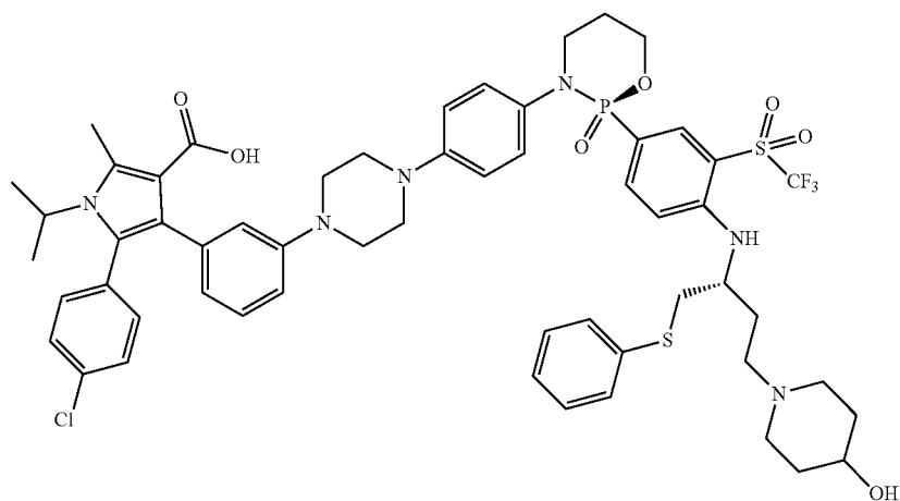
5-(4-chlorophenyl)-4-(3-(4-(4-((R)-2-4-((R)-4-(4-hydroxypiperidin-1-yl)-1-(phenylthio)butan-2-yl)amino)-3-((trifluoromethyl)sulfonyl)phenyl)-2-oxido-1,3,2-oxazaphosphinan-3-yl)phenyl)piperazin-1-yl)phenyl)-1-isopropyl-2-methyl-1H-pyrrole-3-carboxylic acid
