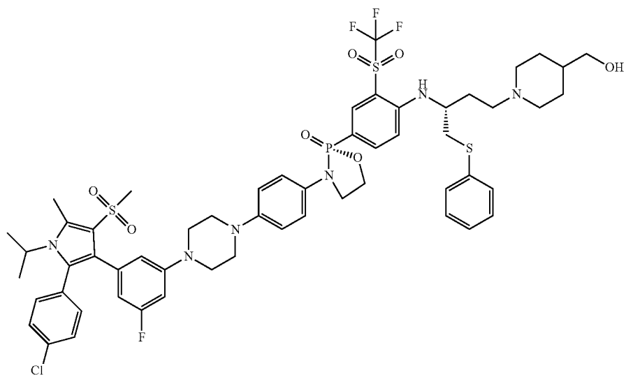
(R)-3-(4-(4-(3-(2-(4-chlorophenyl)-1-isopropyl-5-methyl-4-(methylsulfonyl)-1H-pyrrol-3-yl)-5-fluorophenyl)piperazin-1-yl)phenyl)-2-(4(((R)-4-(4-(hydroxymethyl)piperidin-1-yl)-1-(phenylthio)butan-2-yl)amino)-3-(trifluoromethyl)sulfonyl)phenyl)-1,3,2-oxazaphospholidine 2-oxide
