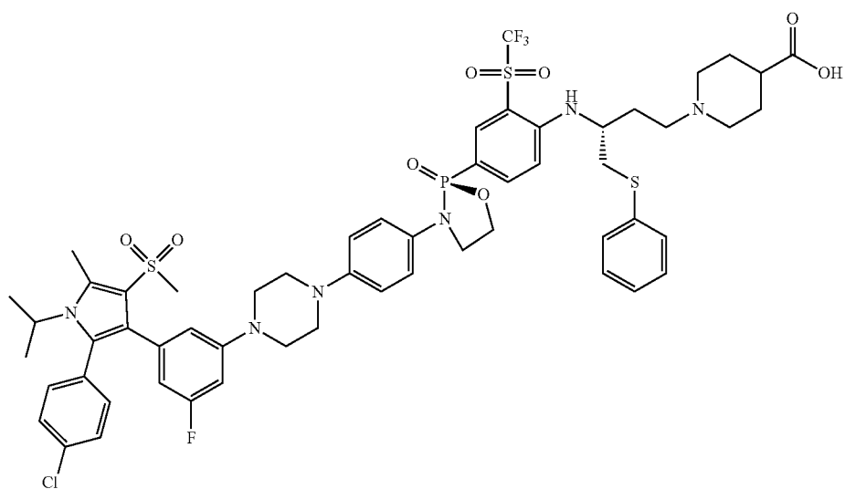
1-((R)-3-((4-((S)-3-(4-(3-(2-(4-chlorophenyl)-1-isopropyl-5-methyl-4-(methylsulfonyl)-1H-pyrrol-3-yl)phenyl)piperazin-1-yl)phenyl)-2-oxido-1,3,2-oxazaphospholidin-2-yl)-2-(trifluoromethyl)sulfonyl)phenyl)amino)-4-(phenylthio)butyl)piperidine-4-carboxylic acid
