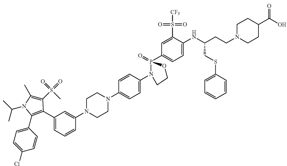
1-((R)-3-((4-((S)-3-(4-(4-(3-(2-(4-chlorophenyl)-1-isopropyl-5-methyl-4-(methylsulfonyl)-1H-pyrrol-3-yl)phenyl)piperazin-1-yl)phenyl)-2-oxido-1,3,2-oxazaphospholidin-2-yl)-2-(trifluoromethyl)sulfonyl)phenyl)amino)-4-(phenylthio)butyl)piperidine-4-carboxylic acid
