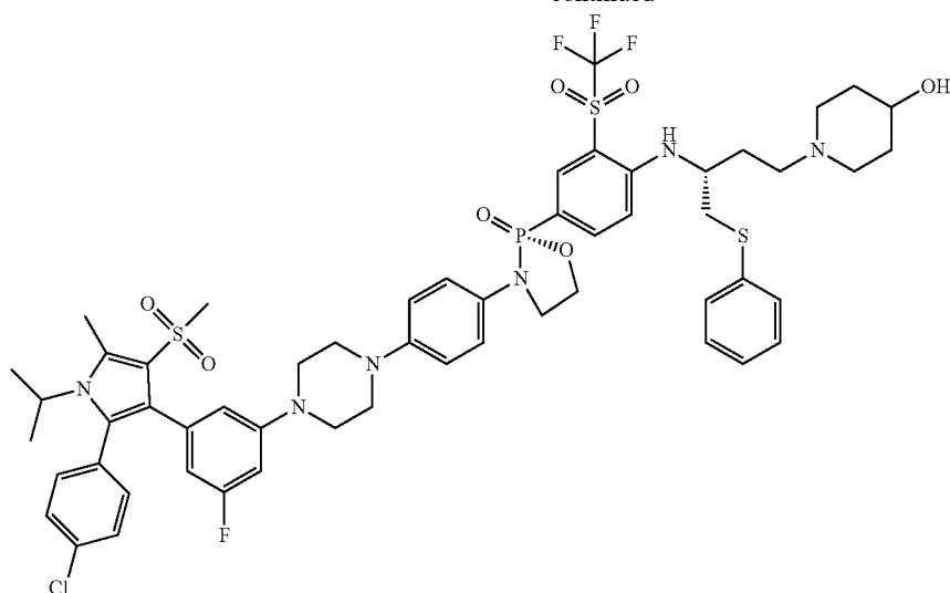
(R)-3-(4-(4-(3-(2-(4-chlorophenyl)-1-isopropyl-5-methyl-4-(methylsulfonyl)-1H-pyrrol-3-yl)-5-fluorophenyl)piperazin-1-yl)phenyl)-2-(4-(((R)-4-(4-hydroxypiperidin-1-yl)-1-(phenylthio)butan-2-yl)amino)-3-(trifluoromethyl)sulfonyl)phenyl)-1,3,2-oxazaphospholidine 2-oxide
