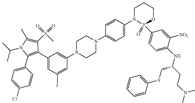
(R)-3-(4-(4-(3-(2-(4-chlorophenyl)-1-isopropyl-5-methyl-4-(methylsulfonyl)-1H-pyrrol-3-yl)-5-fluorophenyl)piperazin-1-yl)phenyl)-2-(4-(((R)-4-(dimethylamino)-1-(phenylthio)butan-2-yl)amino)-3-nitrophenyl)-1,3,2-oxazaphosphinane 2-oxide
