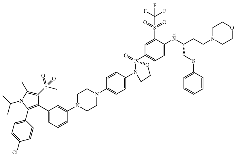
(R)-3-(4-(4-(3-(2-(4-chlorophenyl)-1-isopropyl-5-methyl-4-(methylsulfonyl)-1H-pyrrol-3-yl)phenyl)piperazin-1-yl)phenyl)-2-(4-(((R)-4-morpholino-1-(phenylthio)butan-2-yl)amino)-3-((trifluoromethyl)sulfonyl)phenyl)-1,3,2-oxazaphospholidine 2-oxide
