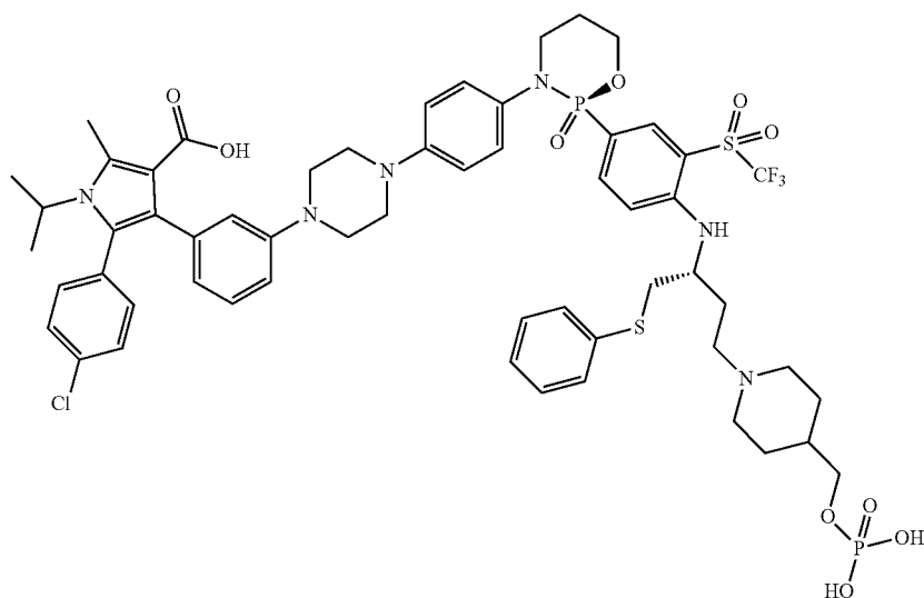
5-(4-chlorophenyl)-1-isopropyl-2-methyl-4-(3-(4-(4-((R)-2-oxido-2-(4-((R)-1-(phenylthio)-4-(4-((phosphonoxy)methyl)piperidin-1-yl)butan-2-yl)amino)-3-(trifluoromethyl)sulfonyl)phenyl)-1,3,2-oxazaphosphinan-3-yl)phenyl)piperazin-1-yl)phenyl)-1H-pyrrole-3-carboxylic acid
