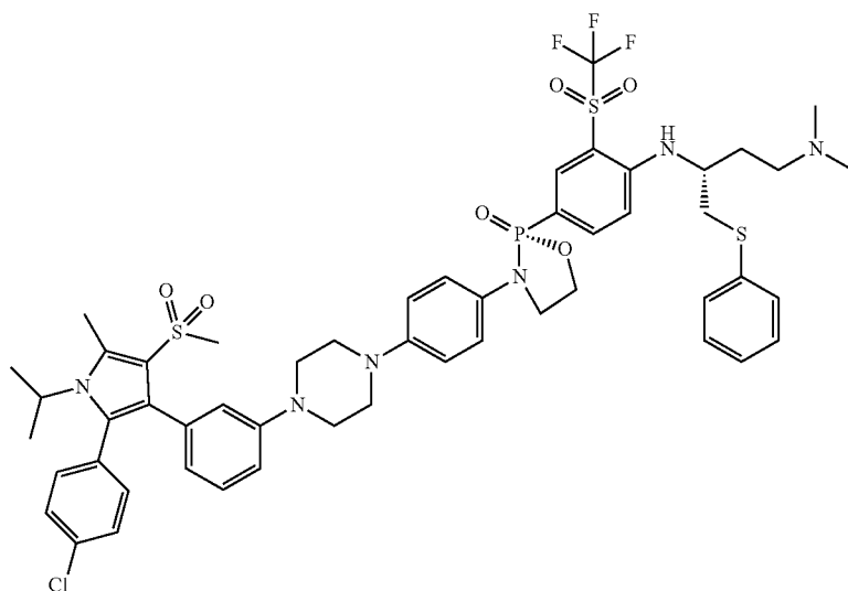
(R)-3-(4-(4-(3-(2-(4-chlorophenyl)-1-isopropyl-5-methyl-4-(methylsulfonyl)-1H-pyrrol-3-yl)phenyl)piperazin-1-yl)phenyl)-2-(4-(((R)-4-(dimethylamino)-1-(phenylthio)butan-2-yl)amino)-3-(trifluoromethyl)sulfonyl)phenyl)-1,3,2-oxazaphospholidine 2-oxide
