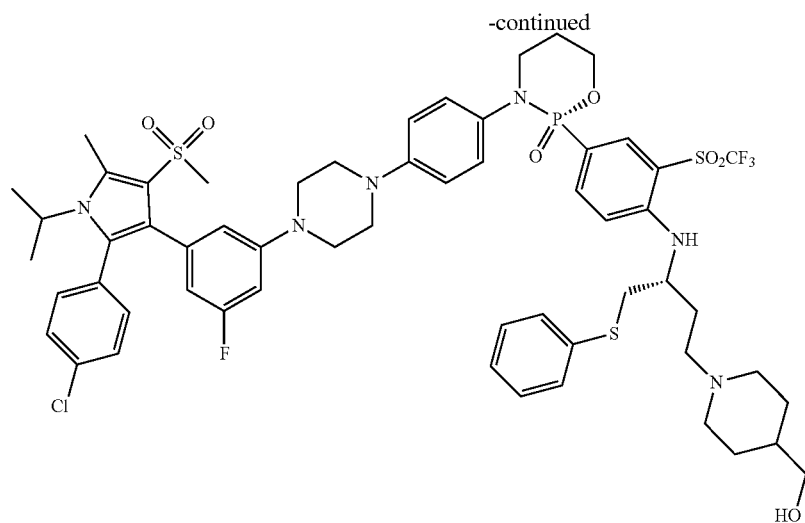
(S)-3-(4-(4-(3-(2-(4-chlorophenyl)-1-isopropyl-5-methyl-4-(methylsulfonyl)-1H-pyrrol-3-yl)-5-fluorophenyl)piperazin-1-yl)phenyl)-2-(4(((R)-4-(4-hydroxymethyl)piperidin-1-yl)-1-(phenylthio)butan-2-yl)amino)-3-(trifluoromethyl)sulfonyl)phenyl)-1,3,2-oxazaphosphinane 2-oxide
