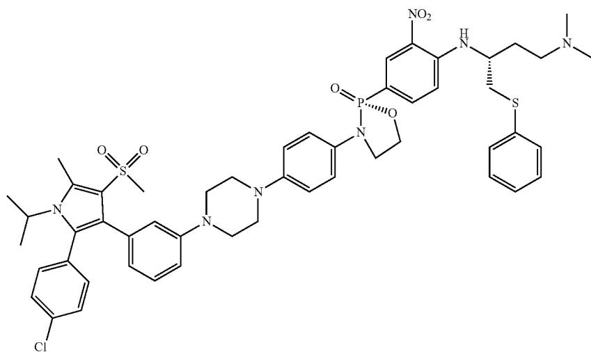
(R)-3-(4-(4-(3-(2-(4-chlorophenyl)-1-isopropyl-5-methyl-4-(methylsulfonyl)-1H-pyrrol-3-yl)phenyl)piperazin-1-yl)phenyl)-2-(4-(((R)-4-(dimethylamino)-1-(phenylthio)butan-2-yl)amino)-3-nitrophenyl)-1,3,2-oxazaphospholidine 2-oxide
