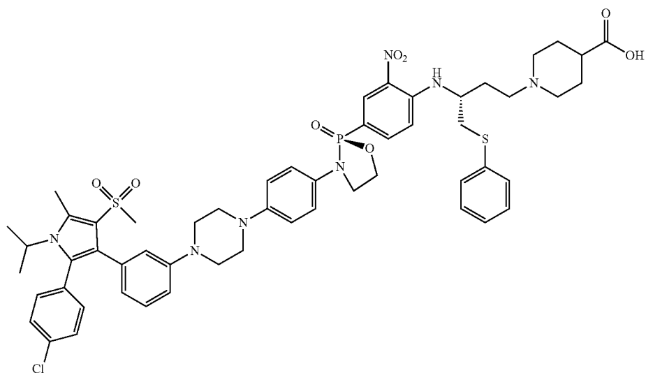
1-((S)-3-((4-((R)-3-(4-(4-(3-(2-(4-chlorophenyl)-1-isopropyl-5-methyl-4-(methylsulfonyl)-1H-pyrrol-3-yl)phenyl)piperazin-1-yl)phenyl)-2-oxido-1,3,2-oxazaphospholidin-2-yl)-2-nitrophenyl)amino)-4-(phenylthio)butyl)piperidine-4-carboxylic acid
