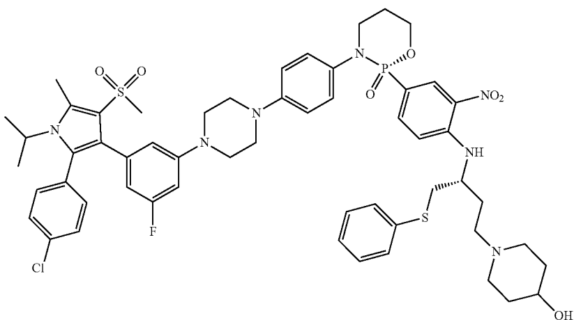
(S)-3-(4-(4-(3-(2-(4-chlorophenyl)-1-isopropyl-5-methyl-4-(methylsulfonyl)-1H-pyrrol-3-yl)-5-fluorophenyl)piperazin-1-yl)phenyl)-2-(4-(((R)-4-(4-hydroxypiperidin-1-yl)-1-(phenylthio)butan-2-yl)amino)-3-nitrophenyl)-1,3,2-oxazaphosphinane 2-oxide
