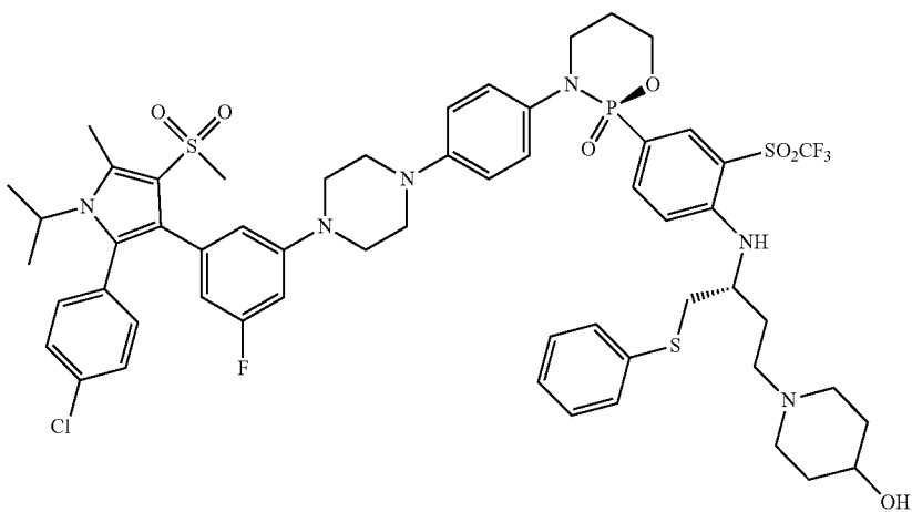
(S)-3-(4-(4-(3-(2-(4-chlorophenyl)-1-isopropyl-5-methyl-4-(methylsulfonyl)-1H-pyrrol-3-yl)-5-fluorophenyl)piperazin-1-yl)phenyl)-2-(4(((R)-4-(dimethylamino)-1-(phenylthio)butan-2-yl)amino)-3-(trifluoromethyl)sulfonyl)phenyl)-1,3,2-oxazaphosphinane 2-oxide
