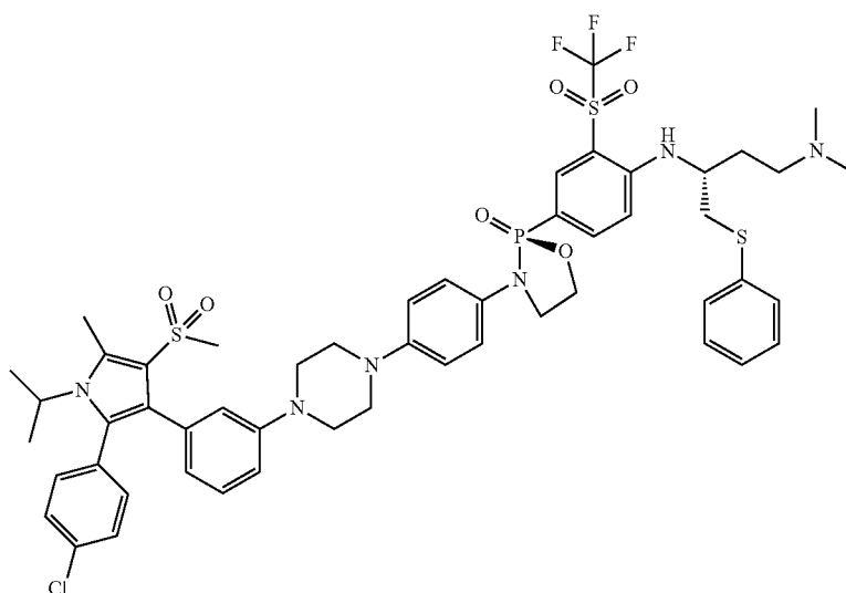
(S)-3-(4-(4-(3-(2-(4-chlorophenyl)-1-isopropyl-5-methyl-4-(methylsulfonyl)-1H-pyrrol-3-yl)phenyl)piperazin-1-yl)phenyl)-2-(4-(((R)-4-(dimethylamino)-1-(phenylthio)butan-2-yl)amino)-3-(trifluoromethyl)sulfonyl)phenyl)-1,3,2-oxazaphospholidine 2-oxide
