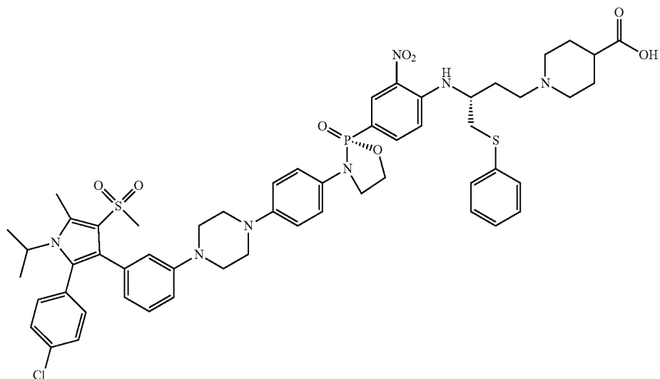
1-((R)-3-((4-((R)-3-(4-(3-(2-(4-chlorophenyl)-1-isopropyl-5-methyl-4-(methylsulfonyl)-1H-pyrrol-3-yl)phenyl)piperazin-1-yl)phenyl)-2-oxido-1,3,2-oxazaphospholidin-2-yl)-2-nitrophenyl)amino)-4-(phenylthio)butyl)piperidine-4-carboxylic acid
