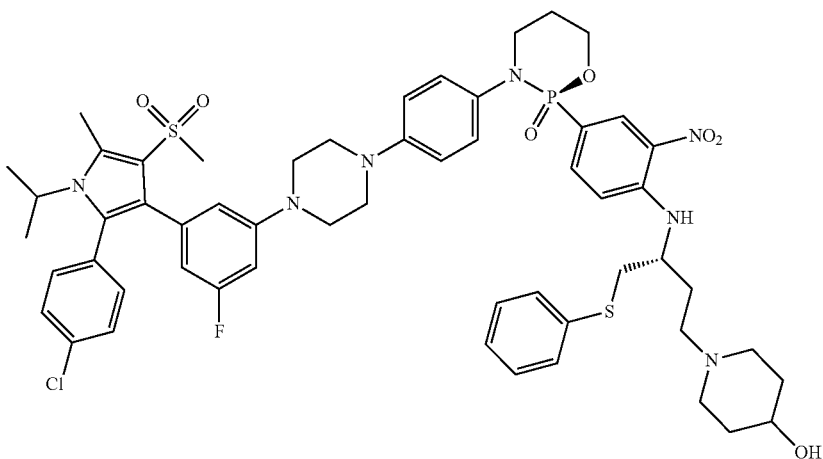
(R)-3-(4-(4-(3-(2-(4-chlorophenyl)-1-isopropyl-5-methyl-4-(methylsulfonyl)-1H-pyrrol-3-yl)-5-fluorophenyl)piperazin-1-yl)phenyl)-2-(4-(((R)-4-(4-hydroxypiperidin-1-yl)-1-(phenylthio)butan-2-yl)amino)-3-nitrophenyl)-1,3,2-oxazaphosphinane 2-oxide
