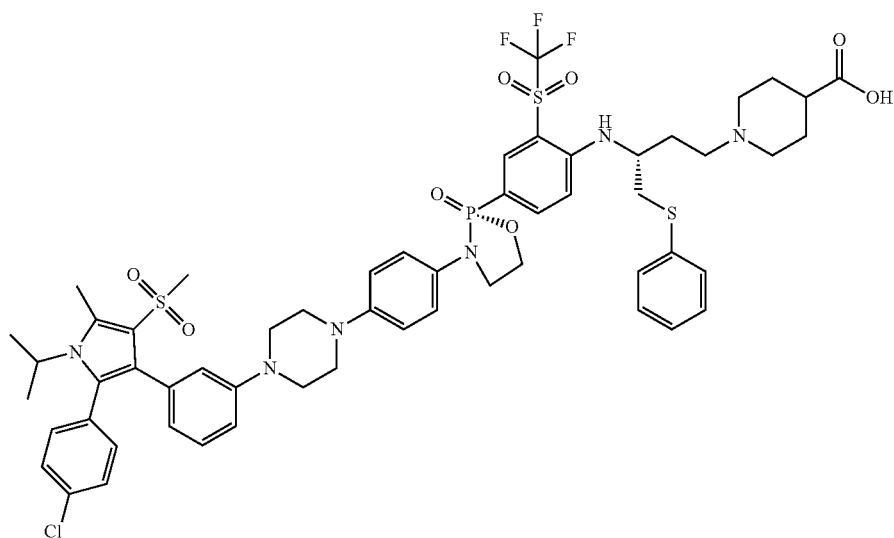
1-((R)-3-(4-((R)-3-(4-(3-(2-(4-chlorophenyl)-1-isopropyl-5-methyl-4-(methylsulfonyl)-1H-pyrrol-3-yl)phenyl)piperazin-1-yl)phenyl)-2-oxido-1,3,2-oxazaphospholidin-2-yl)-2-(trifluoromethyl)sulfonyl)phenyl)amino)-4-(phenylthio)butyl)piperidine-4-carboxylic acid
