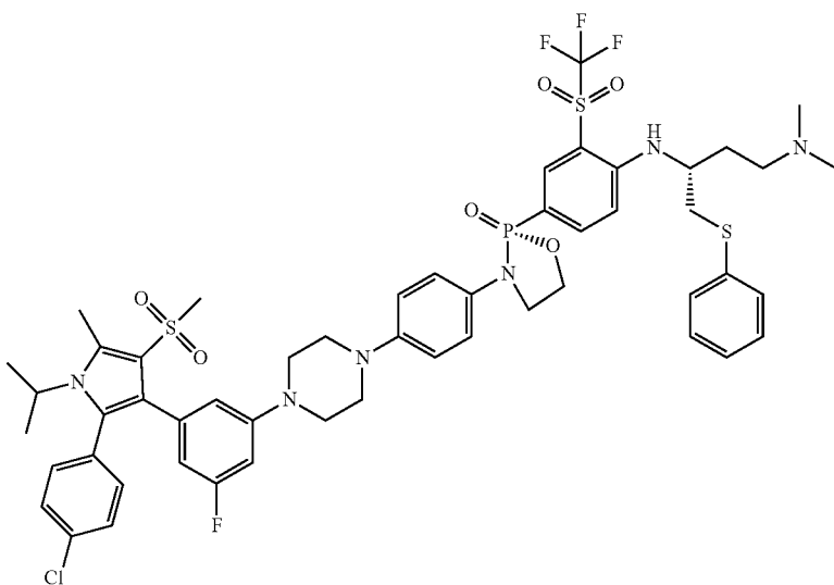
(R)-3-(4-(4-(3-(2-(4-chlorophenyl)-1-isopropyl-5-methyl-4-(methylsulfonyl)-1H-pyrrol-3-yl)-5-fluorophenyl)piperazin-1-yl)phenyl)-2-(4(((R)-4-(dimethylamino)-1-(phenylthio)butan-2-yl)amino)-3-(trifluoromethyl)sulfonyl)phenyl)-1,3,2-oxazaphospholidine 2-oxide
