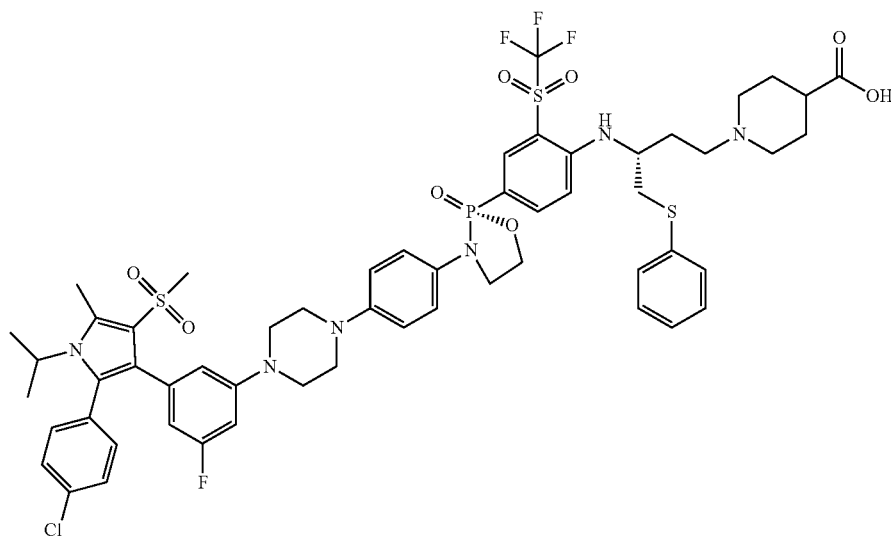
1-((R)-3-((4-((R)-3-(4-(4-(3-(2-(4-chlorophenyl)-1-isopropyl-5-methyl-4-(methylsulfonyl)-1H-pyrrol-3-yl)-5-fluorophenyl)piperazin-1-yl)phenyl)-2-oxido-1,3,2-oxazaphospholidin-2-yl)-2-(trifluoromethyl)sulfonyl)phenyl)amino)-4-(phenylthio)butyl)piperidine-4-carboxylic acid
