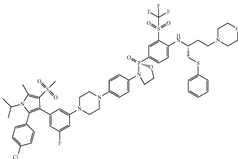
(R)-3-(4-(4-(3-(2-(4-chlorophenyl)-1-isopropyl-5-methyl-4-(methylsulfonyl)-1H-pyrrol-3-yl)-5-fluorophenyl)piperazin-1-yl)phenyl)-2-(4(((R)-4-morpholino-1-(phenylthio)butan-2-yl)amino)-3-(trifluoromethyl)sulfonyl)phenyl)-1,3,2-oxazaphospholidine 2-oxide
