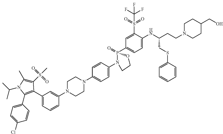
(R)-3-(4-(3-(2-(4-chlorophenyl)-1-isopropyl-5-methyl-4-(methylsulfonyl)-1H-pyrrol-3-yl)phenyl)piperazin-1-yl)phenyl)-2-(4-(((R)-4-(4-(hydroxymethyl)piperidin-1-yl)-1-(phenylthio)butan-2-yl)amino)-3-(trifluoromethyl)sulfonyl)phenyl)-1,3,2-oxazaphospholidine 2-oxide
