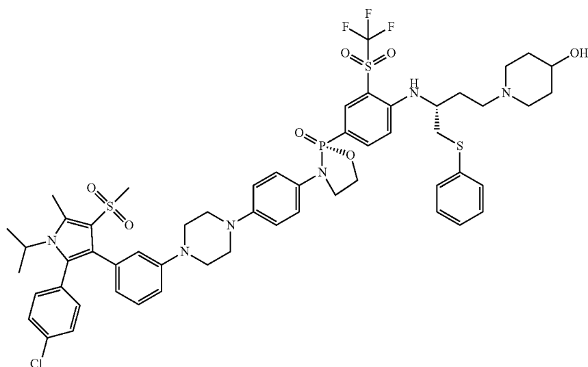
(R)-3-(4-(4-(3-(2-(4-chlorophenyl)-1-isopropyl-5-methyl-4-(methylsulfonyl)-1H-pyrrol-3-yl)phenyl)piperazin-1-yl)phenyl)-2-((R)-4-(4-(hydroxypiperidin-1-yl)-1-(phenylthio)butan-2-yl)amino)-3-(trifluoromethyl)sulfonyl)phenyl)-1,3,2-oxazaphospholidine 2-oxide
