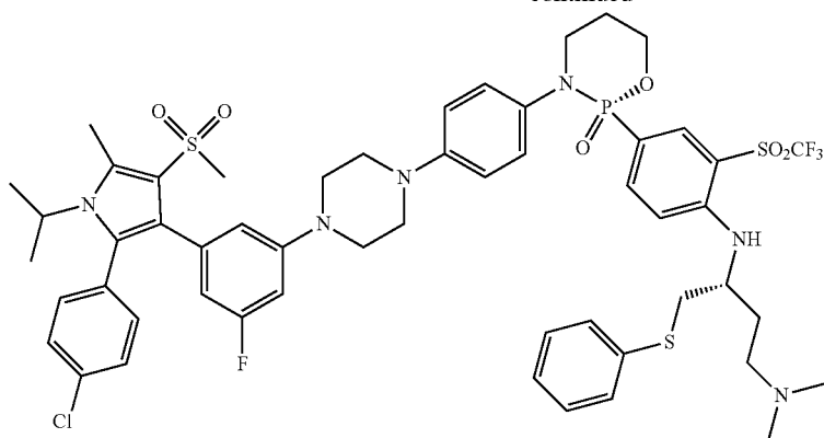
(S)-3-(4-(4-(3-(2-(4-chlorophenyl)-1-isopropyl-5-methyl-4-(methylsulfonyl)-1H-pyrrol-3-yl)-5-fluorophenyl)piperazin-1-yl)phenyl)-2-(4(((R)-4-(dimethylamino)-1-(phenylthio)butan-2-yl)amino)-3-(trifluoromethyl)sulfonyl)phenyl)-1,3,2-oxazaphosphinane 2-oxide
