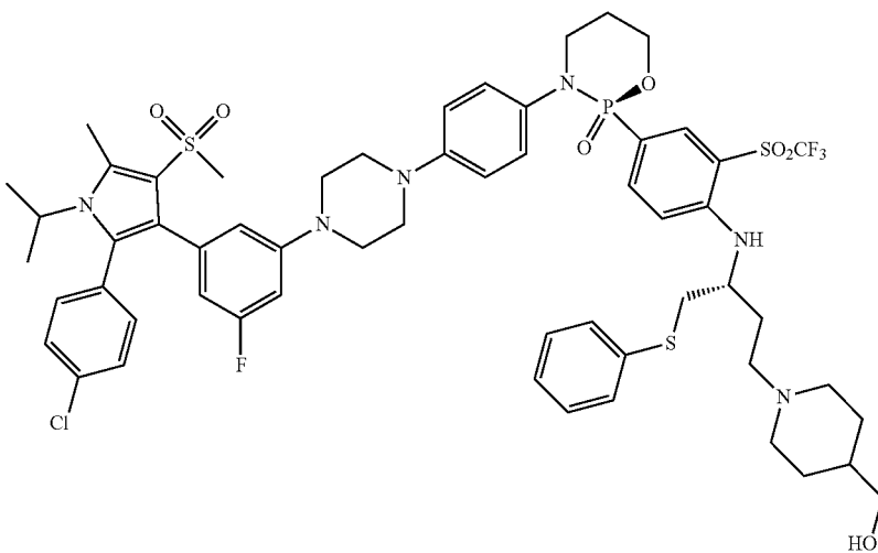
(R)-3-(4-(4-(3-(2-(4-chlorophenyl)-1-isopropyl-5-methyl-4-(methylsulfonyl)-1H-pyrrol-3-yl)-5-fluorophenyl)piperazin-1-yl)phenyl)-2-(4(((R)-4-(4-hydroxymethyl)piperidin-1-yl)-1-(phenylthio)butan-2-yl)amino)-3-(trifluoromethyl)sulfonyl)phenyl)-1,3,2-oxazaphosphinane 2-oxide
