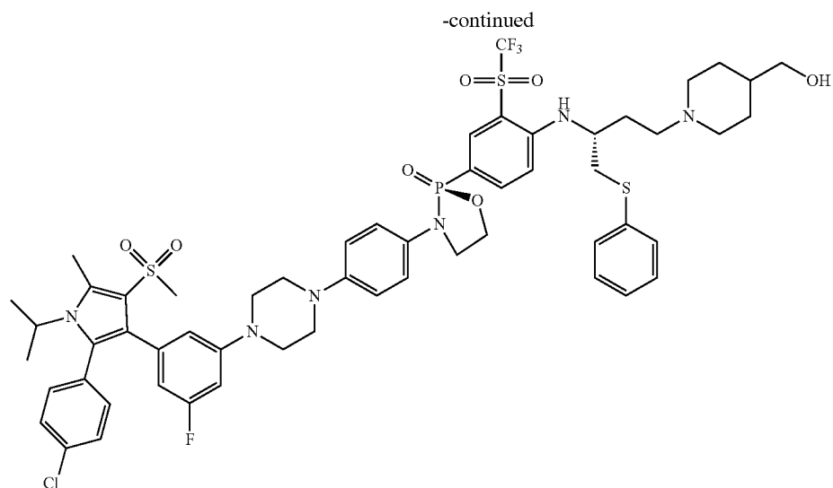
(S)-3-(4-(4-(3-(2-(4-chlorophenyl)-1-isopropyl-5-methyl-4-(methylsulfonyl)-1H-pyrrol-3-yl)-5-fluorophenyl)piperazin-1-yl)phenyl)-2-(((R)-4-(4-hydroxymethyl)piperidin-1-yl)-1-(phenylthio)butan-2-yl)amino)-3-(trifluoromethyl)sulfonylphenyl)-1,3,2-oxazaphospholidine 2-oxide
