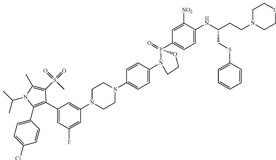
(R)-3-(4-(4-(3-(2-(4-chlorophenyl)-1-isopropyl-5-methyl-4-(methylsulfonyl)-1H-pyrrol-3-yl)-5-fluorophenyl)piperazin-1-yl)phenyl)-2-(4-(((R)-4-morpholino-1-(phenylthio)butan-2-yl)amino)-3-nitrophenyl)-1,3,2-oxazaphospholidine 2-oxide
