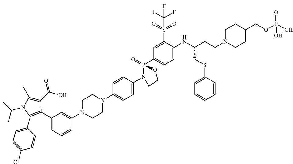
5-(4-chlorophenyl)-1-isopropyl-2-methyl-4-(3-(4-(4-((S)-2-oxido-2-4-(((R)-1-(phenylthio)-4-(4-((phosphonoxy)methyl)piperidin-1-yl)butan-2-yl)amino)-3-(trifluoromethyl)sulfonyl)phenyl)-1,3,2-oxazaphospholidin-3-yl)phenyl)piperazin-1-yl)phenyl)-1H-pyrrole-3-carboxylic acid
