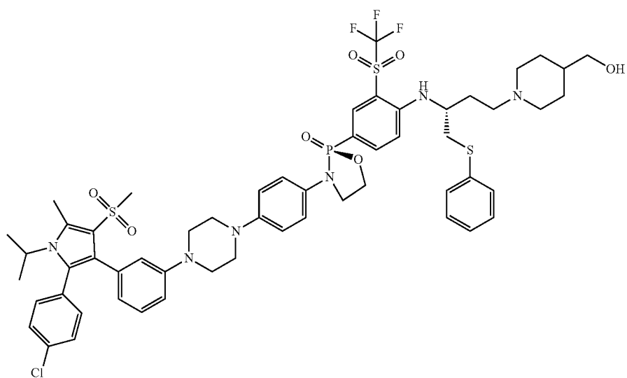
(S)-3-(4-(4-(3-(2-(4-chlorophenyl)-1-isopropyl-5-methyl-4-(methylsulfonyl)-1H-pyrrol-3-yl)phenyl)piperazin-1-yl)phenyl)-2-(4-(((R)-4-(4-(hydroxymethyl)piperidin-1-yl)-1-(phenylthio)butan-2-yl)amino)-3-(trifluoromethyl)sulfonyl)phenyl)-1,3,2-oxazaphospholidine 2-oxide
