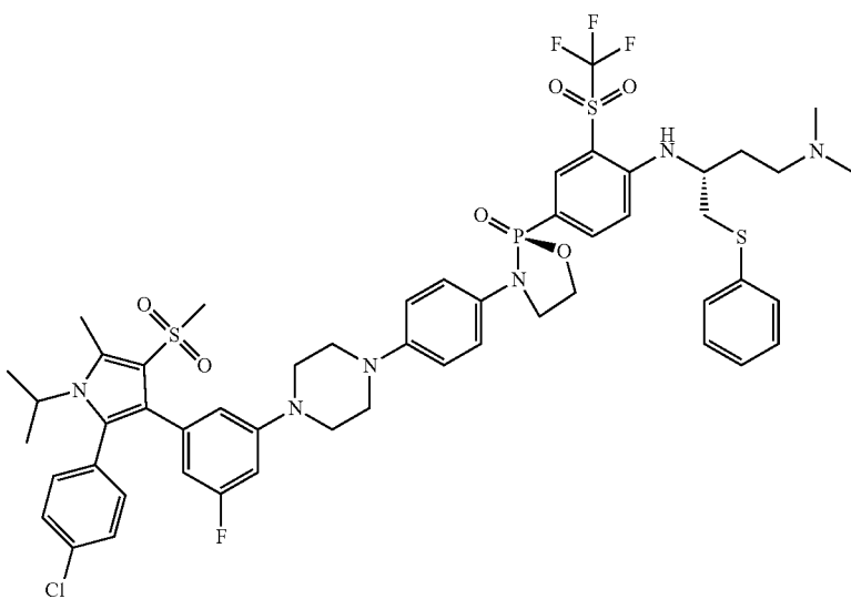
(S)-3-(4-(4-(3-(2-(4-chlorophenyl)-1-isopropyl-5-methyl-4-(methylsulfonyl)-1H-pyrrol-3-yl)-5-fluorophenyl)piperazin-1-yl)phenyl)-2-(4(((R)-4-(dimethylamino)-1-(phenylthio)butan-2-yl)amino)-3-(trifluoromethyl)sulfonyl)phenyl)-1,3,2-oxazaphospholidine 2-oxide
