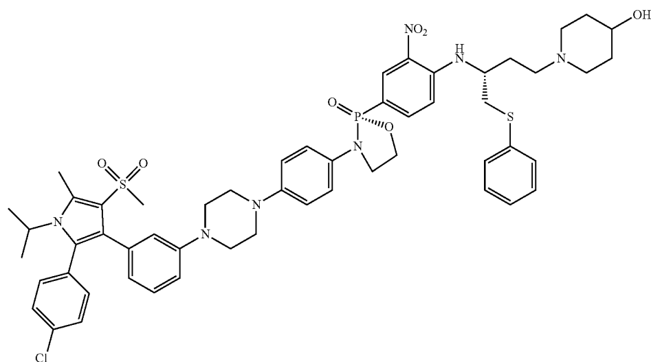
(R)-3-(4-(4-(3-(2-(4-chlorophenyl)-1-isopropyl-5-methyl-4-(methylsulfonyl)-1H-pyrrol-3-yl)-phenyl)piperazin-1-yl)phenyl)-2-(((R)-4-(4-hydroxypiperidin-1-yl)-1-(phenylthio)butan-2-yl)amino)-3-nitrophenyl)-1,3,2-oxazaphospholidine 2-oxide
