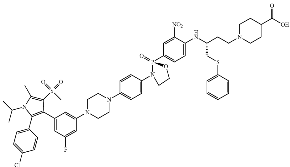
1-((R)-3-((S)-3-(4-(4-(3-(2-(4-chlorophenyl)-1-isopropyl-5-methyl-4-(methylsulfonyl)-1H-pyrrol-3-yl)-5-fluorophenyl)piperazin-1-yl)phenyl)-2-oxido-1,3,2-oxazaphospholidin-2-yl)-2-nitrophenyl)amino)-4-(phenylthio)butyl)piperidine-4-carboxylic acid
