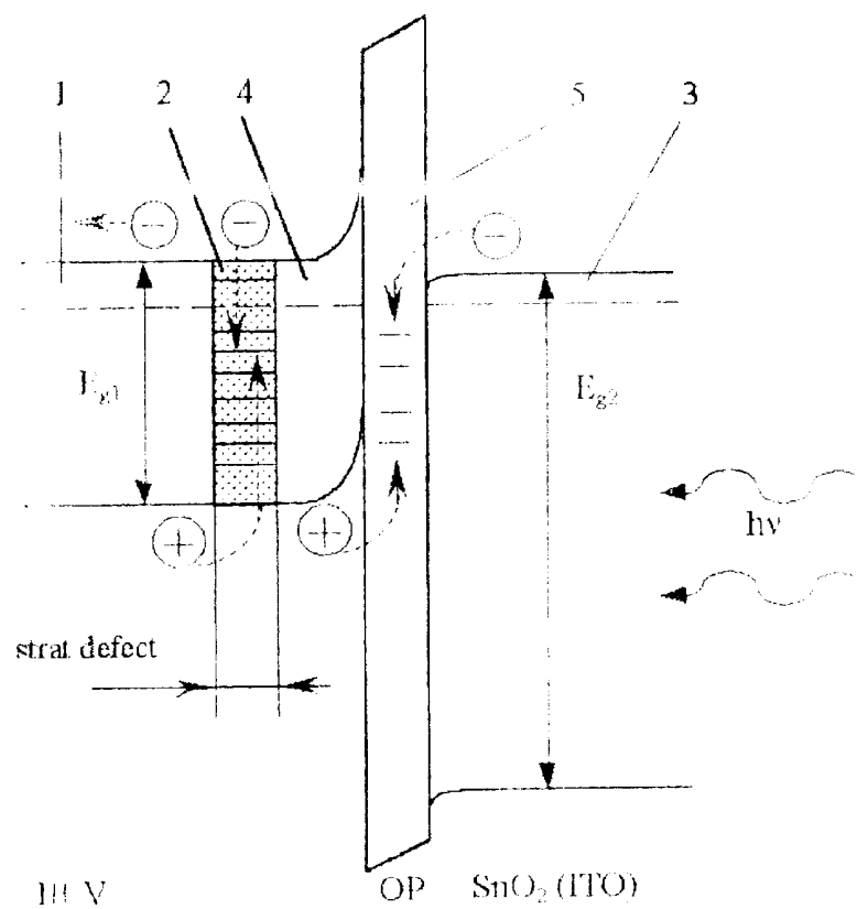
1 - semiconductor cu bandă energetică E_{g1} ; 2 - strat defect; 3 - semiconductor cu bandă energetică E_{g2} ; 4 - strat de sarcină spațială; 5 - oxid propriu.
