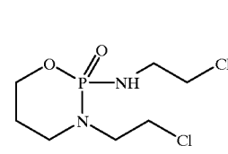
Ifosfamide
