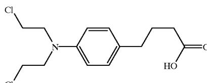
Chlorambucil
