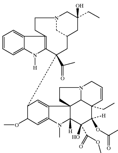
Vinblastine
