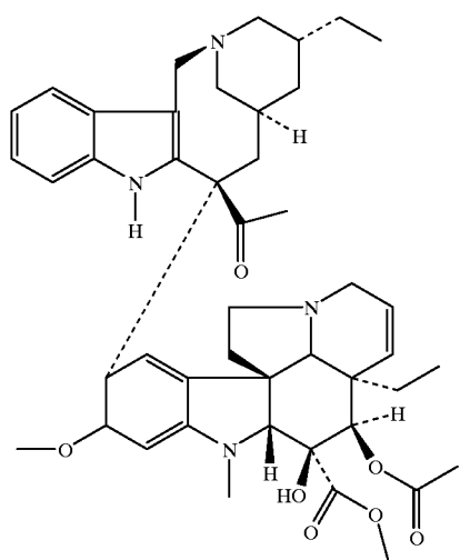
Vinorelbine
