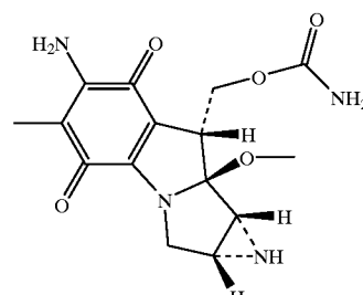
Mitomycin
