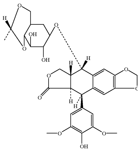
Etoposide
