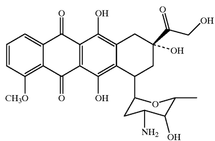
Doxorubicin
