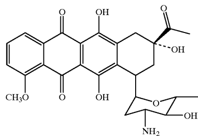
Epirubicin
