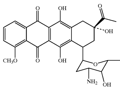
Daunorubicin
