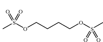
Busulfan
