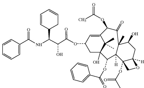
Taxol
