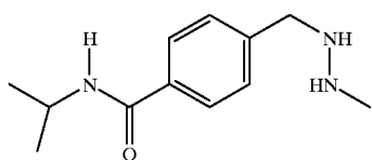
Procarbazine
