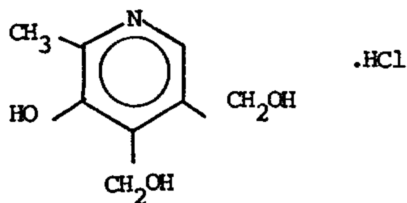
Pyridoxine HCl
