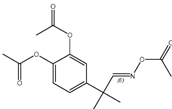
4-(1-(Acetoxyimino)-2-methylpropan-2-yl)-1,2-phenylendiacetat Verbindung 12
