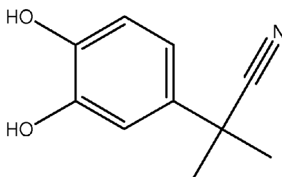
2-(3,4-Dihydroxyphenyl)-2-methylpropanitril Verbindung 10
