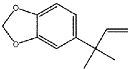
5-(2-méthyl-but-3-én-2-yl)benzo[d][1,3]dioxole Composé 14
