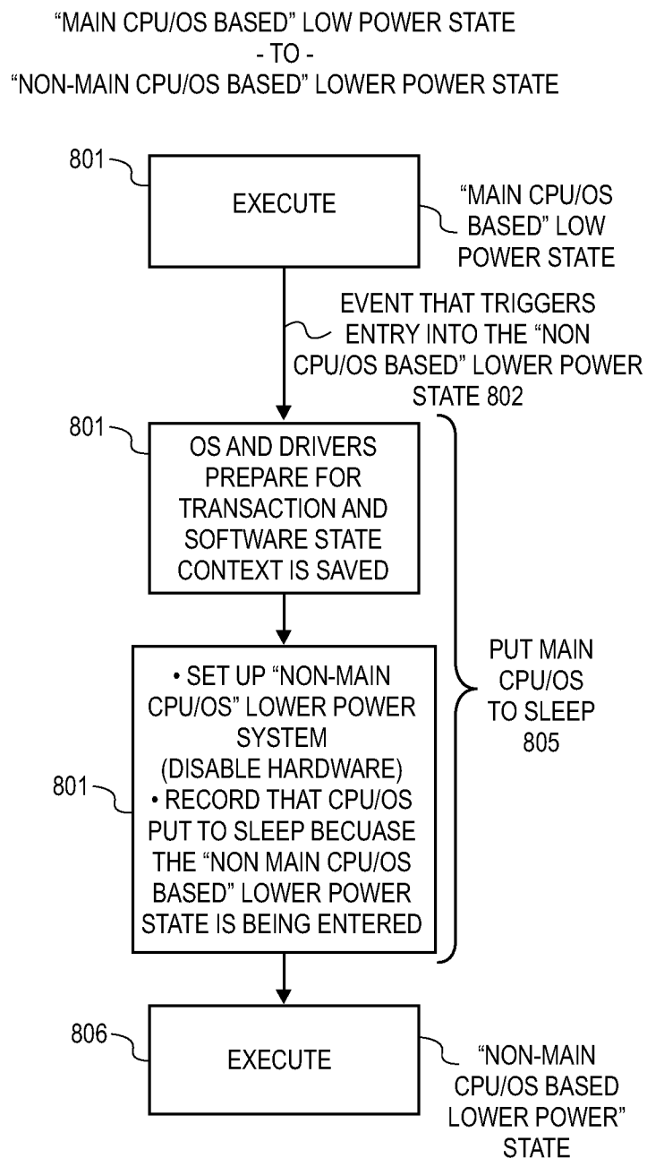
FIG. 8A
