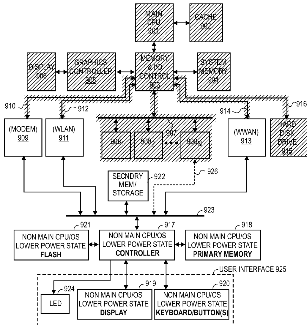
FIG. 9A
