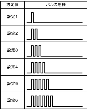
設定変更対応信号 (パルス態様)
