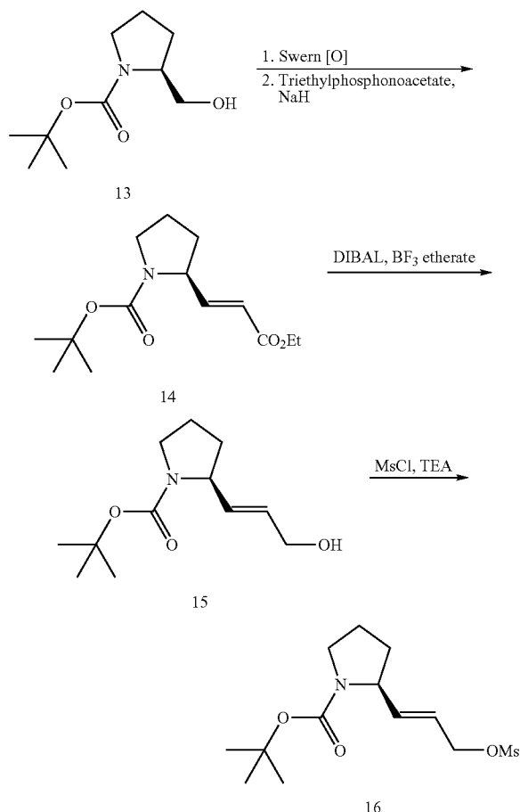
Scheme VI
