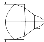
実施例7の断面図と波長 \lambda = 650 \text{ nm} に対する光路図
