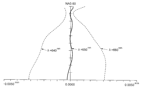
実施例6の波長 \lambda = 650 \pm 10 \text{ nm} に対する球面収差図
