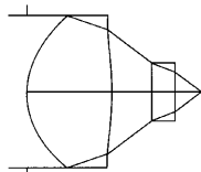
実施例6の断面図と波長 \lambda = 650 \text{ nm} に対する光路図
