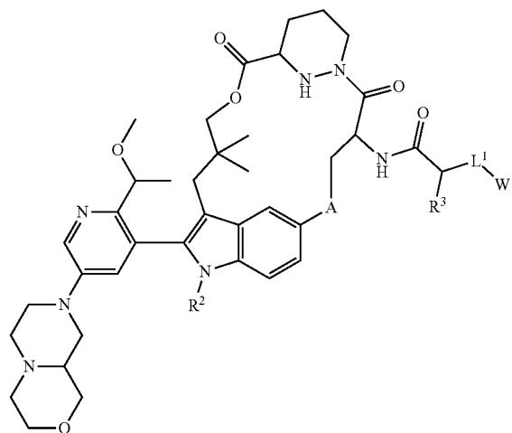
Formula II-4b
