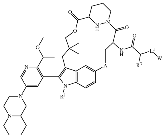
Formula II-4
