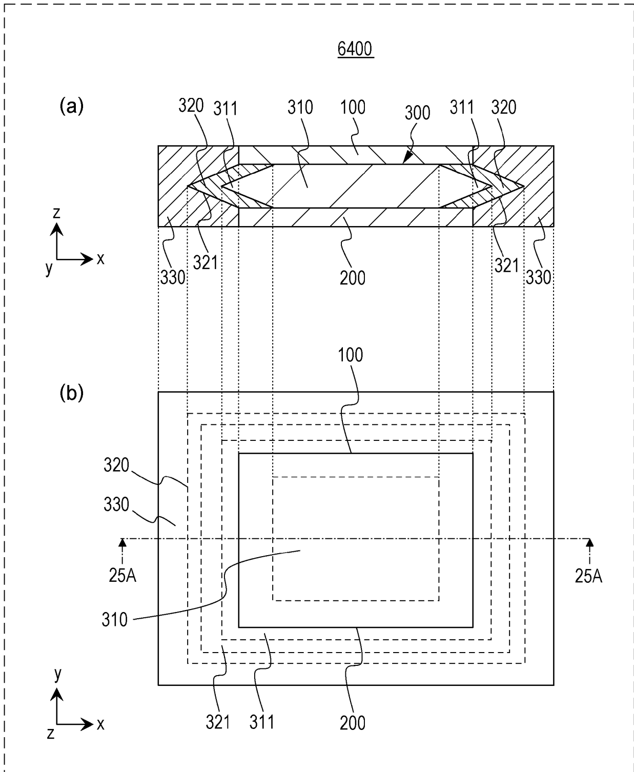
FIG. 25
