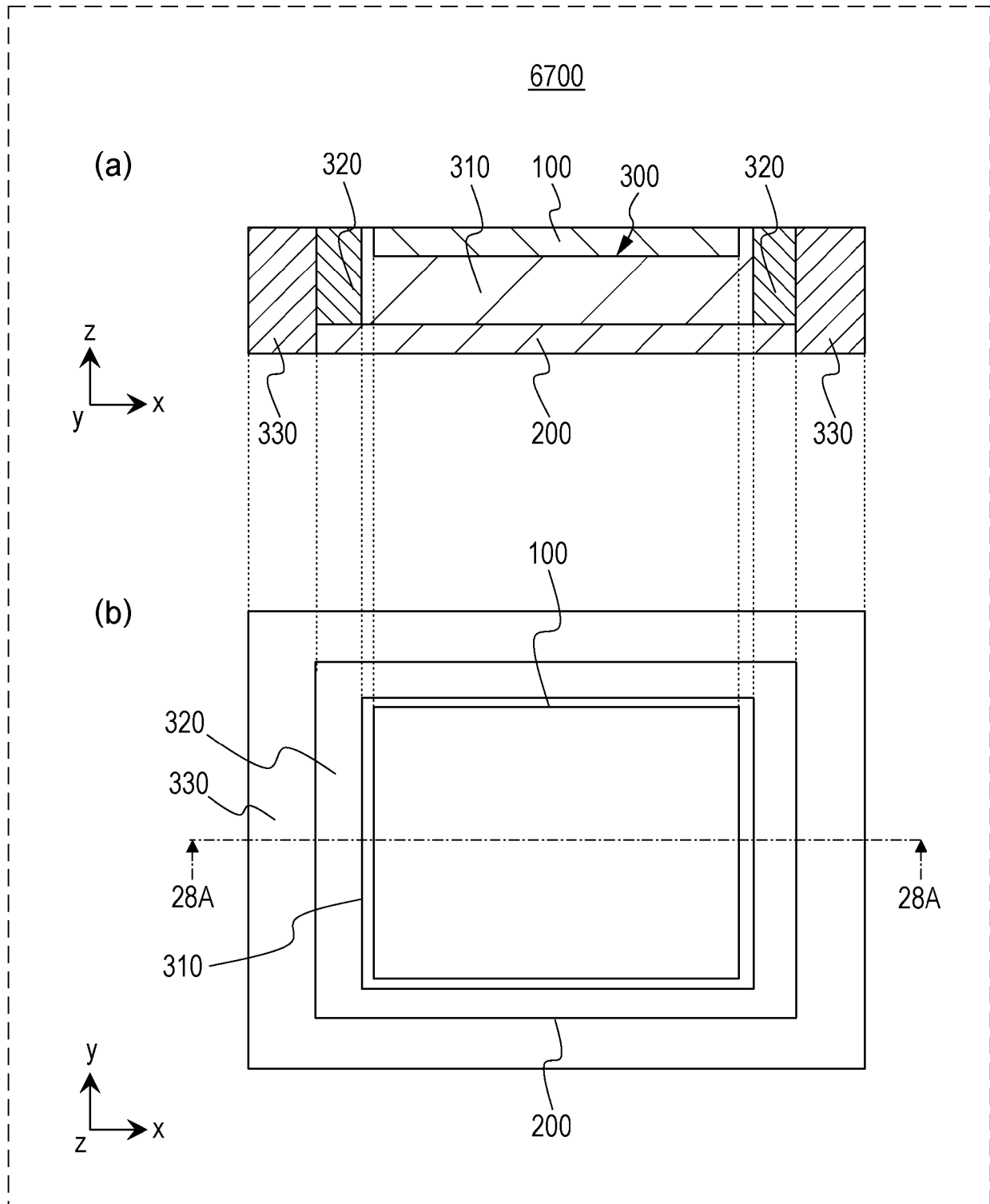
FIG. 28
