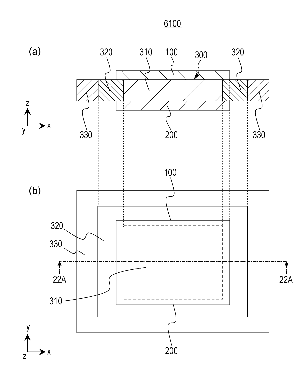
FIG. 22
