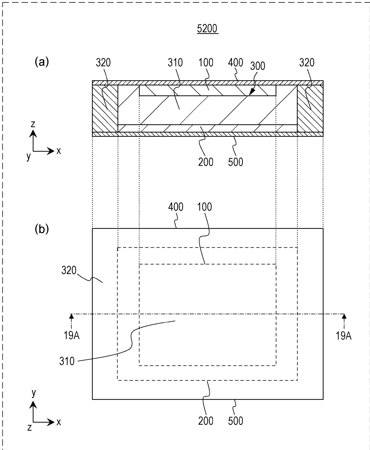
FIG. 19
