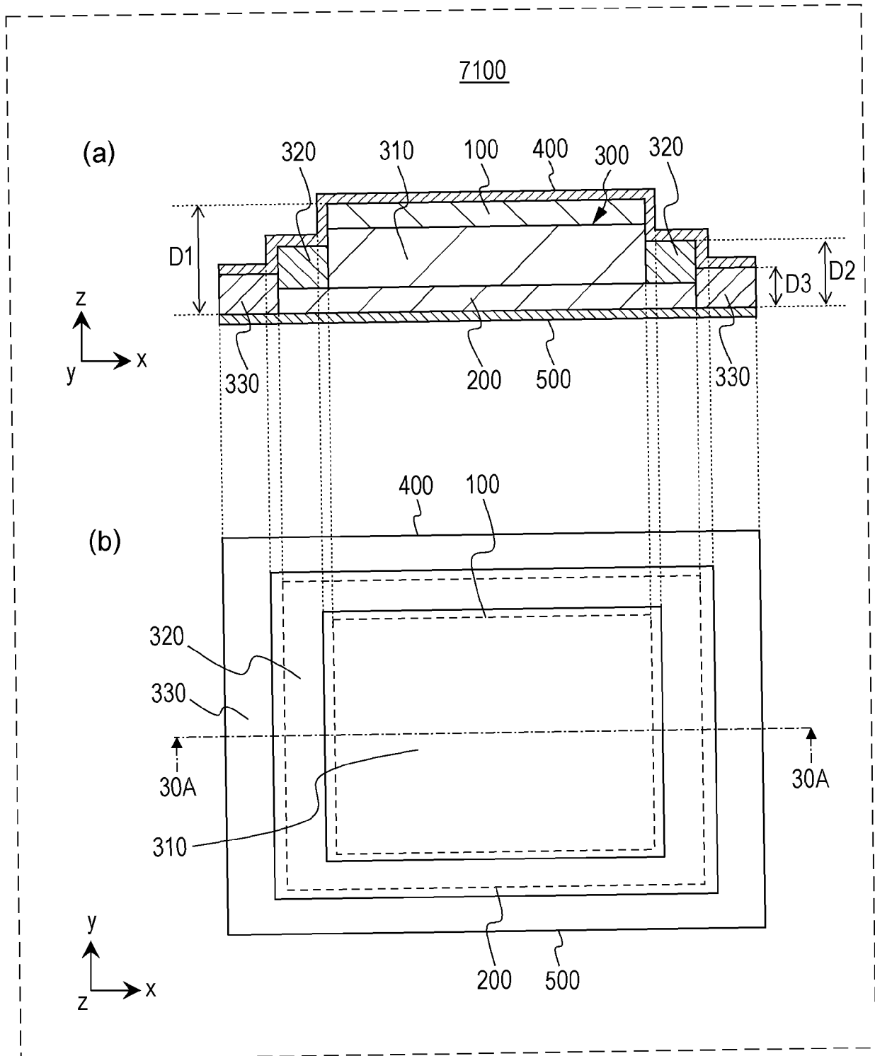
FIG. 30
