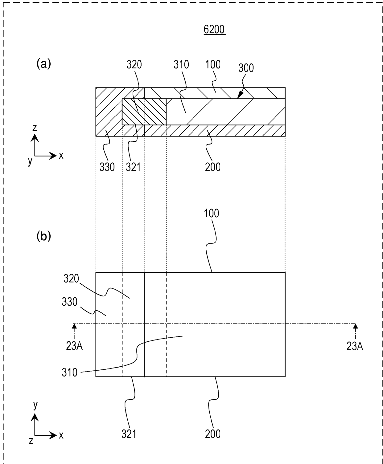
FIG. 23
