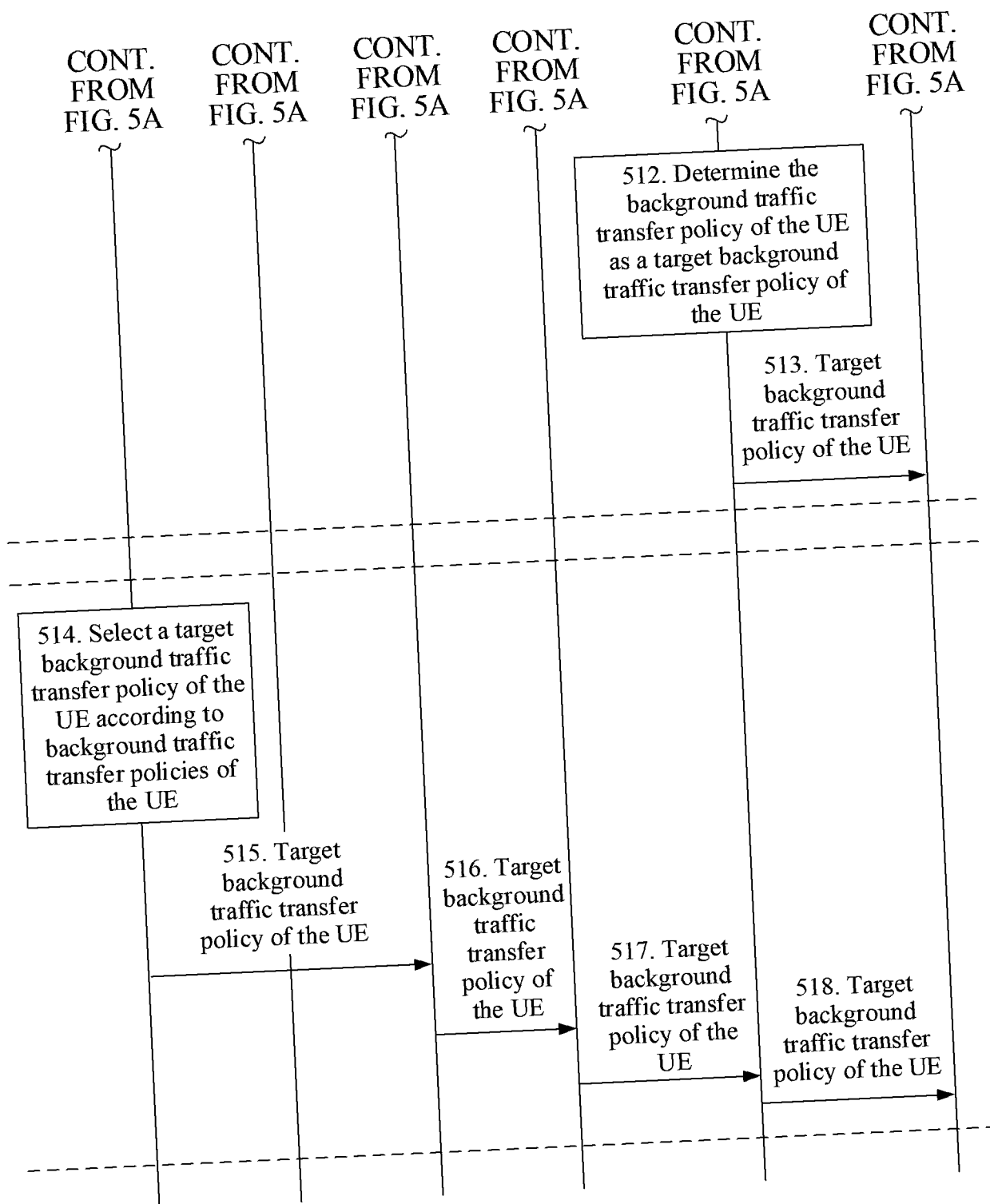
FIG. 5B
