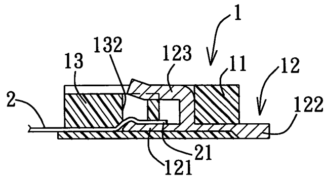
F I G. 3 PRIOR ART
