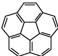
Corannulene
