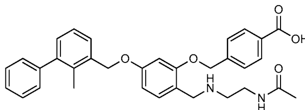
Example 1044: N-(2-((2-ethoxy-4-((2-methyl-[1,1'-biphenyl]-3-yl)methoxy)benzyl)amino)ethyl)acetamide
