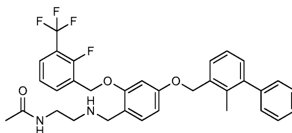
Example 1080: N-(2-((2-((2-fluoro-5-(trifluoromethyl)benzyl)oxy)-4-((2-methyl-[1,1'-biphenyl]-3-yl)methoxy)benzyl)amino)ethyl)acetamide
