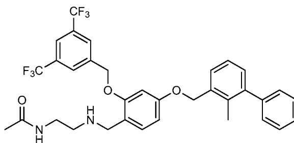
Example 1062: N-(2-((2-((3,5-difluorobenzyl)oxy)-4-((2-methyl-[1,1'-biphenyl]-3-yl)methoxy)benzyl)amino)ethyl)acetamide
