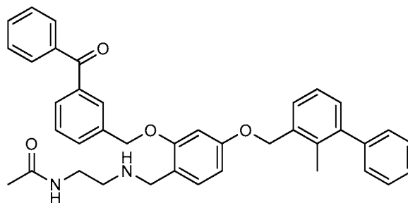
Example 1074: N-(2-((4-((2-methyl-[1,1'-biphenyl]-3-yl)methoxy)-2-(quinolin-8-ylmethoxy)benzyl)amino)ethyl)acetamide
