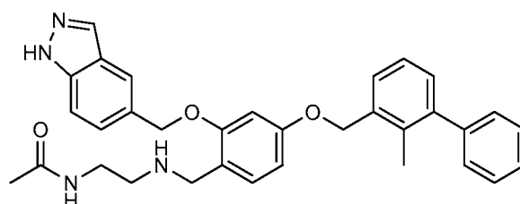
Example 1099: N-(2-((4-((2-methyl-[1,1'-biphenyl]-3-yl)methoxy)-2-((1-(tetrahydro-2H-pyran-2-yl)-1H-indazol-5-yl)methoxy)benzyl)amino)ethyl)acetamide
