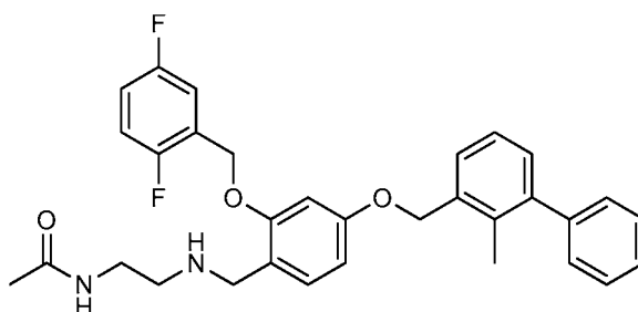
Example 1061: N-(2-((2-((3,5-bis(trifluoromethyl)benzyl)oxy)-4-((2-methyl-[1,1'-biphenyl]-3-yl)methoxy)benzyl)amino)ethyl)acetamide
