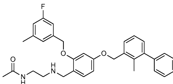
Example 1114: N-(2-((2-((3-cyano-4-fluorobenzyl)oxy)-4-((2-methyl-[1,1'-biphenyl]-3-yl)methoxy)benzyl)amino)ethyl)acetamide
