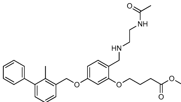
Example 1037: N-(2-((2-((3-(hydroxymethyl)benzyl)oxy)-4-((2-methyl-[1,1'-biphenyl]-3-yl)methoxy)benzyl)amino)ethyl)acetamide
