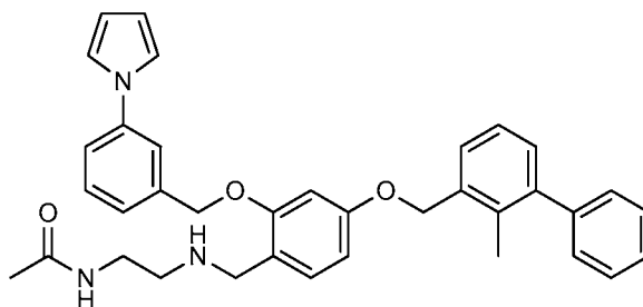
Example 1113: N-(2-((2-((3-fluoro-5-methylbenzyl)oxy)-4-((2-methyl-[1,1'-biphenyl]-3-yl)methoxy)benzyl)amino)ethyl)acetamide
