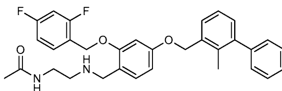
Example 1065: N-(2-((2-((3,5-dimethylbenzyl)oxy)-4-((2-methyl-[1,1'-biphenyl]-3-yl)methoxy)benzyl)amino)ethyl)acetamide
