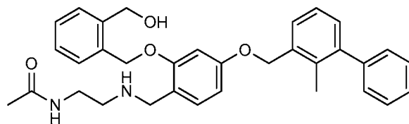
Example 1039: 4-((2-(((2-acetamidoethyl)amino)methyl)-5-((2-methyl-[1,1'-biphenyl]-3-yl)methoxy)phenoxy)methyl)benzamide
