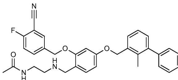
Example 1115: N-(2-((4-((2-methyl-[1,1'-biphenyl]-3-yl)methoxy)-2-((5-methylisoxazol-3-yl)methoxy)benzyl)amino)ethyl)acetamide
