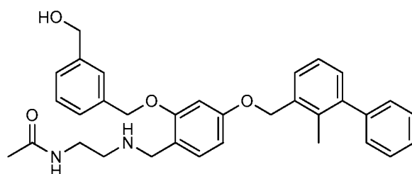
Example 1038: N-(2-((2-((2-(hydroxymethyl)benzyl)oxy)-4-((2-methyl-[1,1'-biphenyl]-3-yl)methoxy)benzyl)amino)ethyl)acetamide
