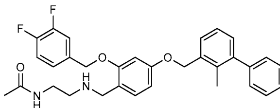
Example 1060: N-(2-((2-((2,5-difluorobenzyl)oxy)-4-((2-methyl-[1,1'-biphenyl]-3-yl)methoxy)benzyl)amino)ethyl)acetamide
