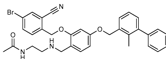
Example 1098: N-(2-((2-((1H-indazol-5-yl)methoxy)-4-((2-methyl-[1,1'-biphenyl]-3-yl)methoxy)benzyl)amino)ethyl)acetamide
