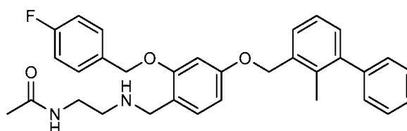
Example 1076: N-(2-((4-((2-methyl-[1,1'-biphenyl]-3-yl)methoxy)-2-((3-nitrobenzyl)oxy)benzyl)amino)ethyl)acetamide
