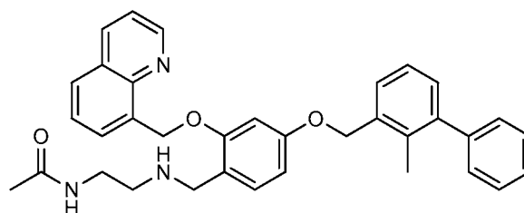
Example 1075: N-(2-((2-((4-fluorobenzyl)oxy)-4-((2-methyl-[1,1'-biphenyl]-3-yl)methoxy)benzyl)amino)ethyl)acetamide
