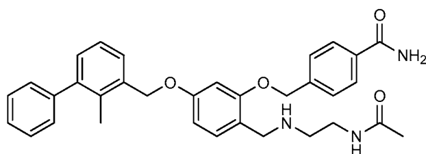
Example 1040: N-(2-((2-((4-acetylbenzyl)oxy)-4-((2-methyl-[1,1'-biphenyl]-3-yl)methoxy)benzyl)amino)ethyl)acetamide
