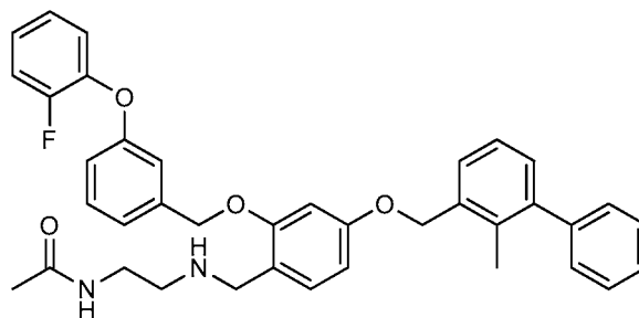
Example 1078: N-(2-((2-((3-(4-fluorophenoxy)benzyl)oxy)-4-((2-methyl-[1,1'-biphenyl]-3-yl)methoxy)benzyl)amino)ethyl)acetamide
