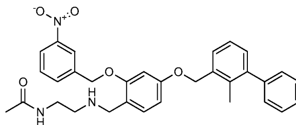
Example 1077: N-(2-((2-((3-(2-fluorophenoxy)benzyl)oxy)-4-((2-methyl-[1,1'-biphenyl]-3-yl)methoxy)benzyl)amino)ethyl)acetamide
