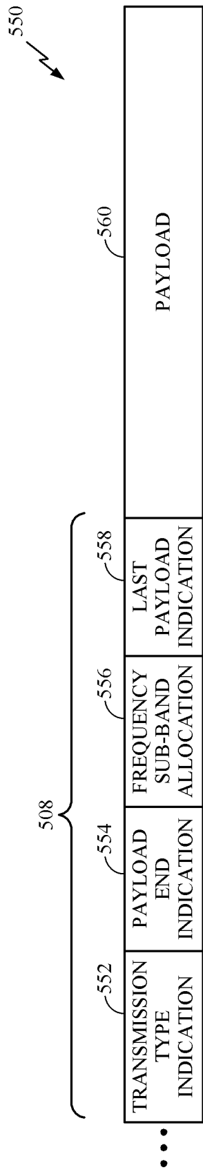
FIG. 5E
