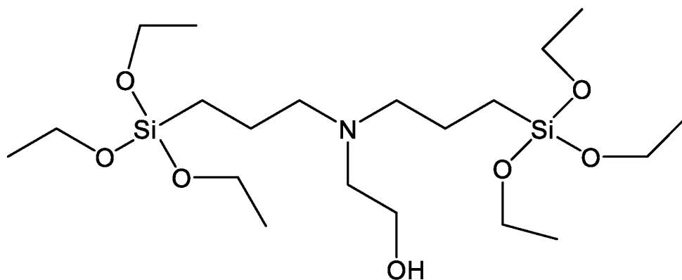
- 2-[Bis[3-(triethoxysilyl)propyl]amino]-ethanol
