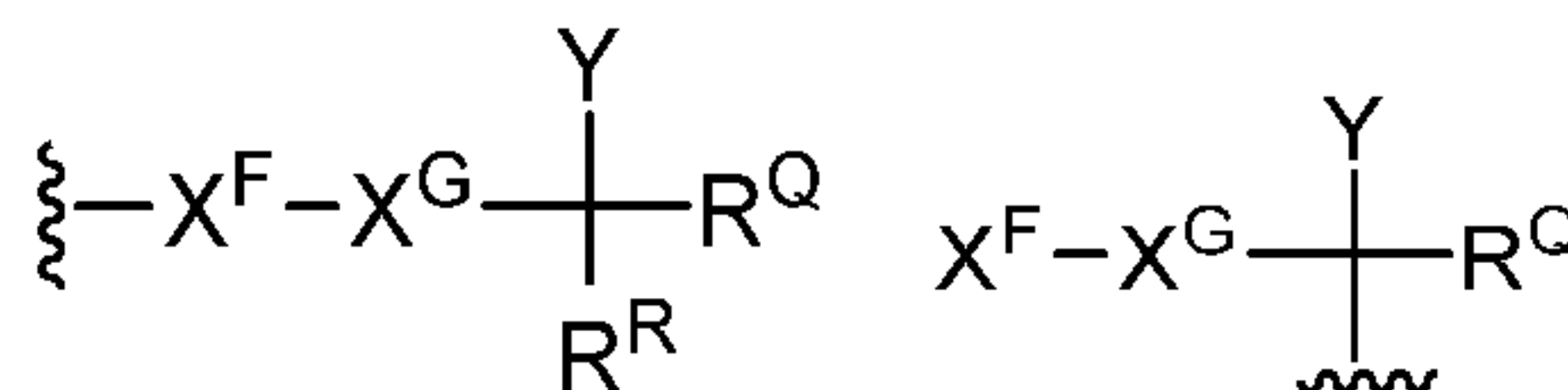
Formula Im
