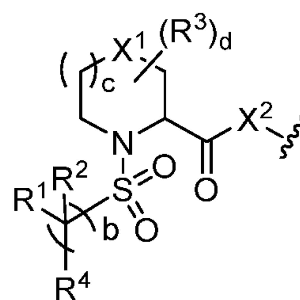
Formula VIIb
