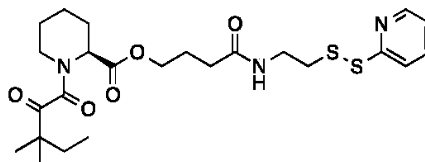
C2Holt
