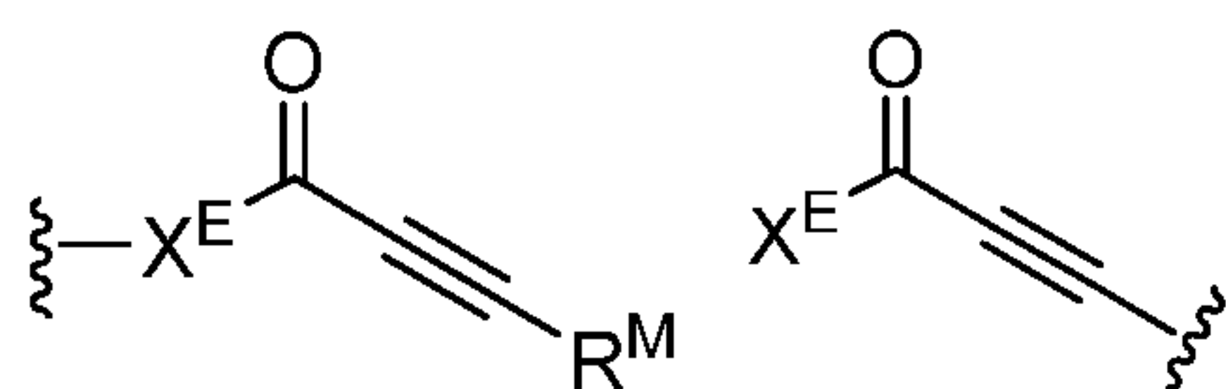
Formula Ij
