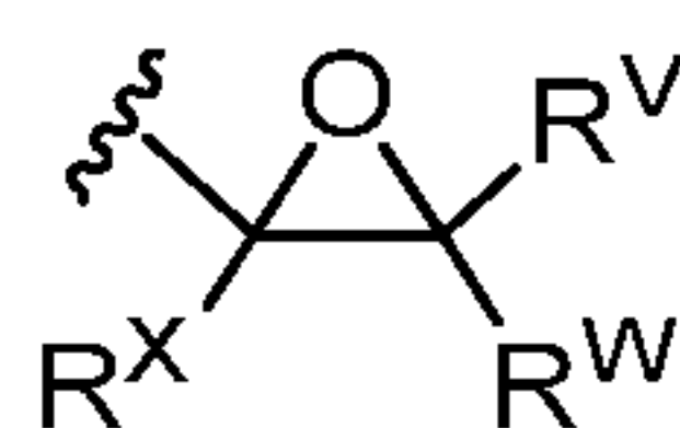
Formula Io
