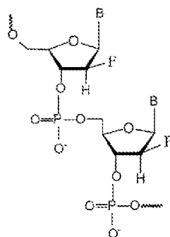
2'-F
