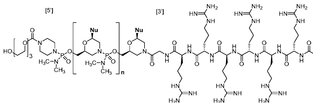
(III)
