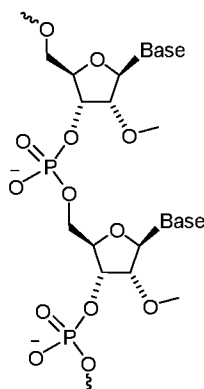
2'-O-Me
