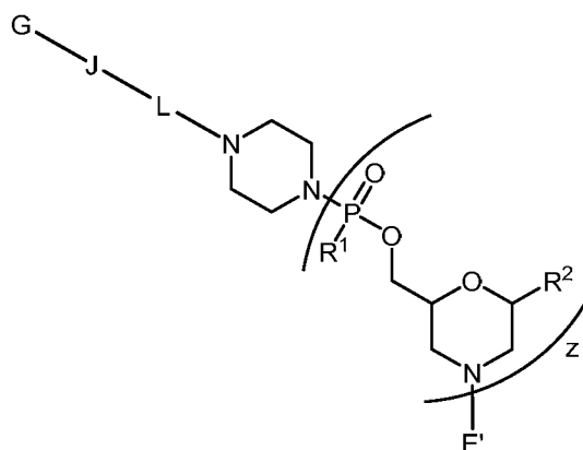
(IVb)
