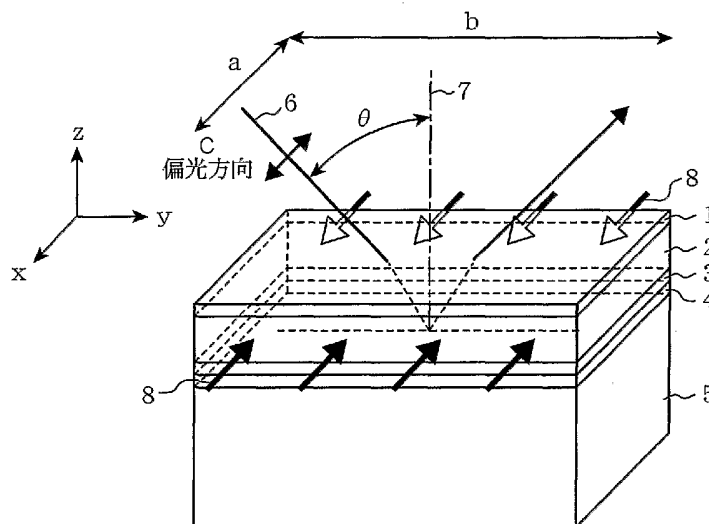
C...POLARIZING DIRECTION
