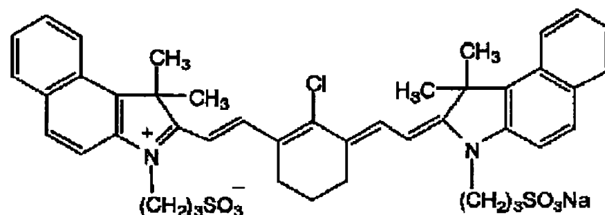
( IR-9 )
