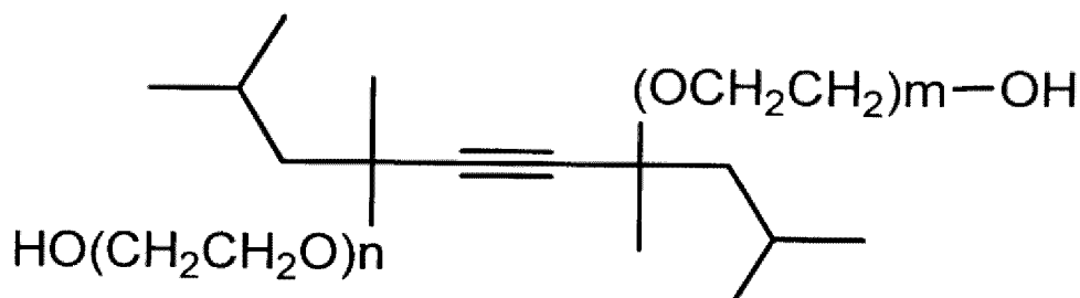
SURFYNOL 465
