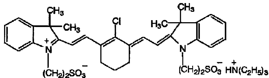
( IR-8 )
