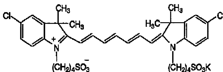
( IR-2 )
