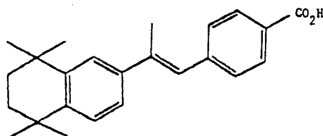
TTNPB
