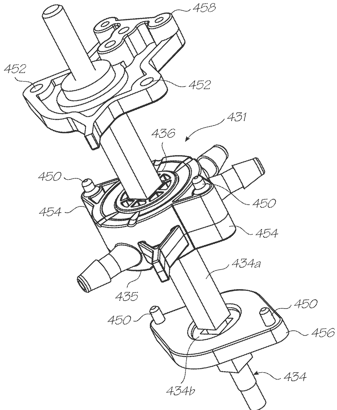
FIG. 32B
