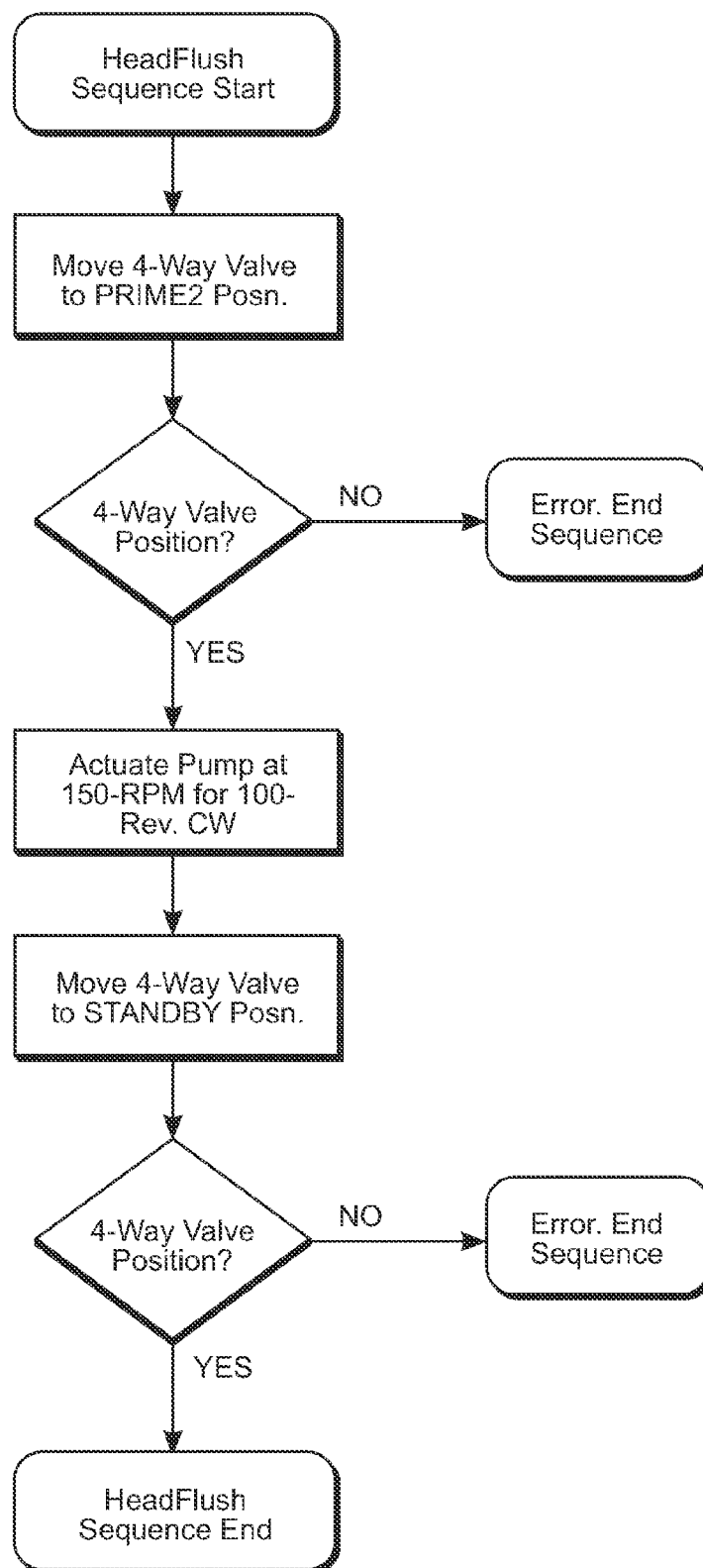
FIG. 22
