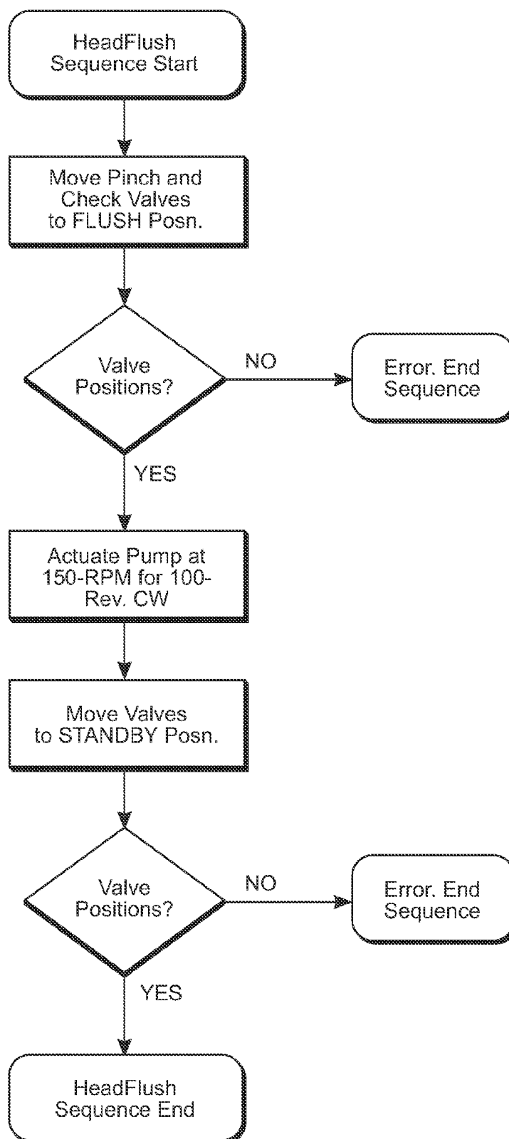
FIG. 45
