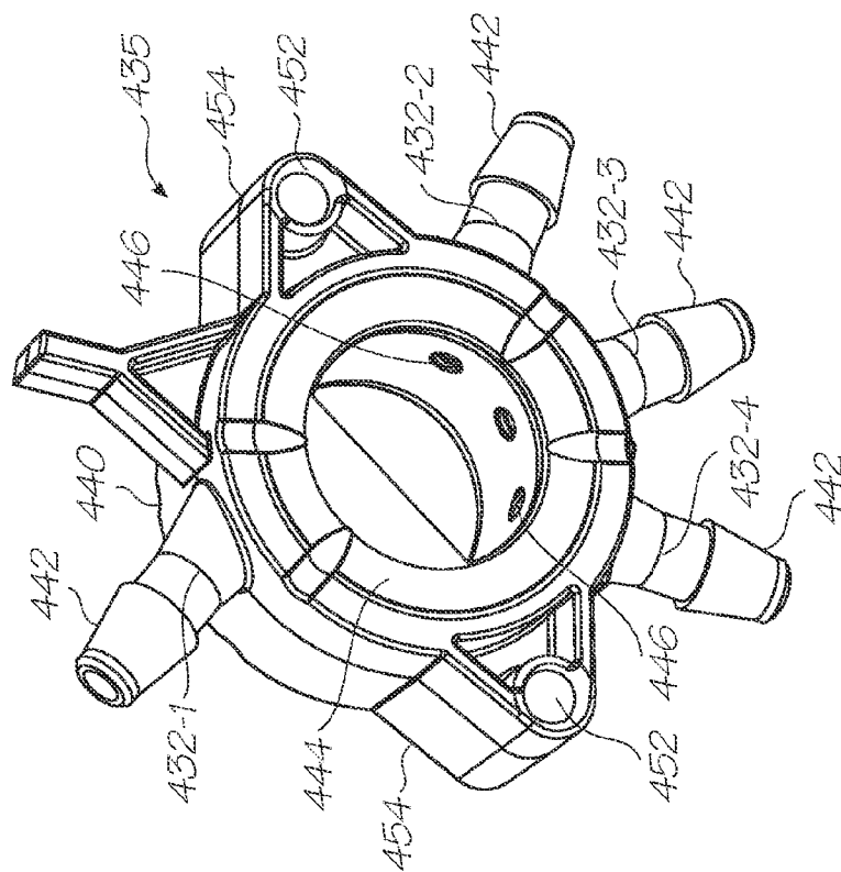
FIG. 33A
