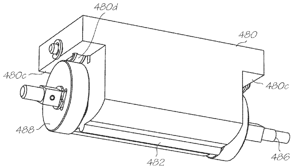
FIG. 42B
