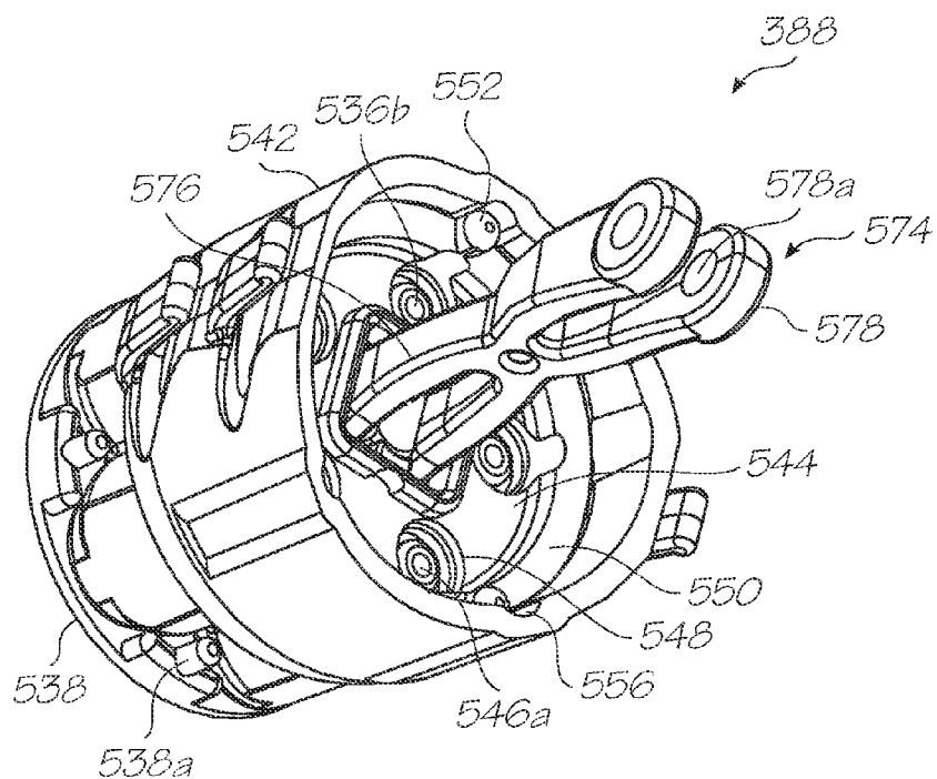
FIG. 53B
