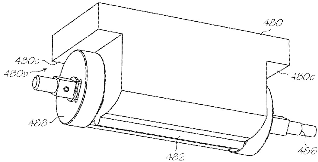
FIG. 42A
