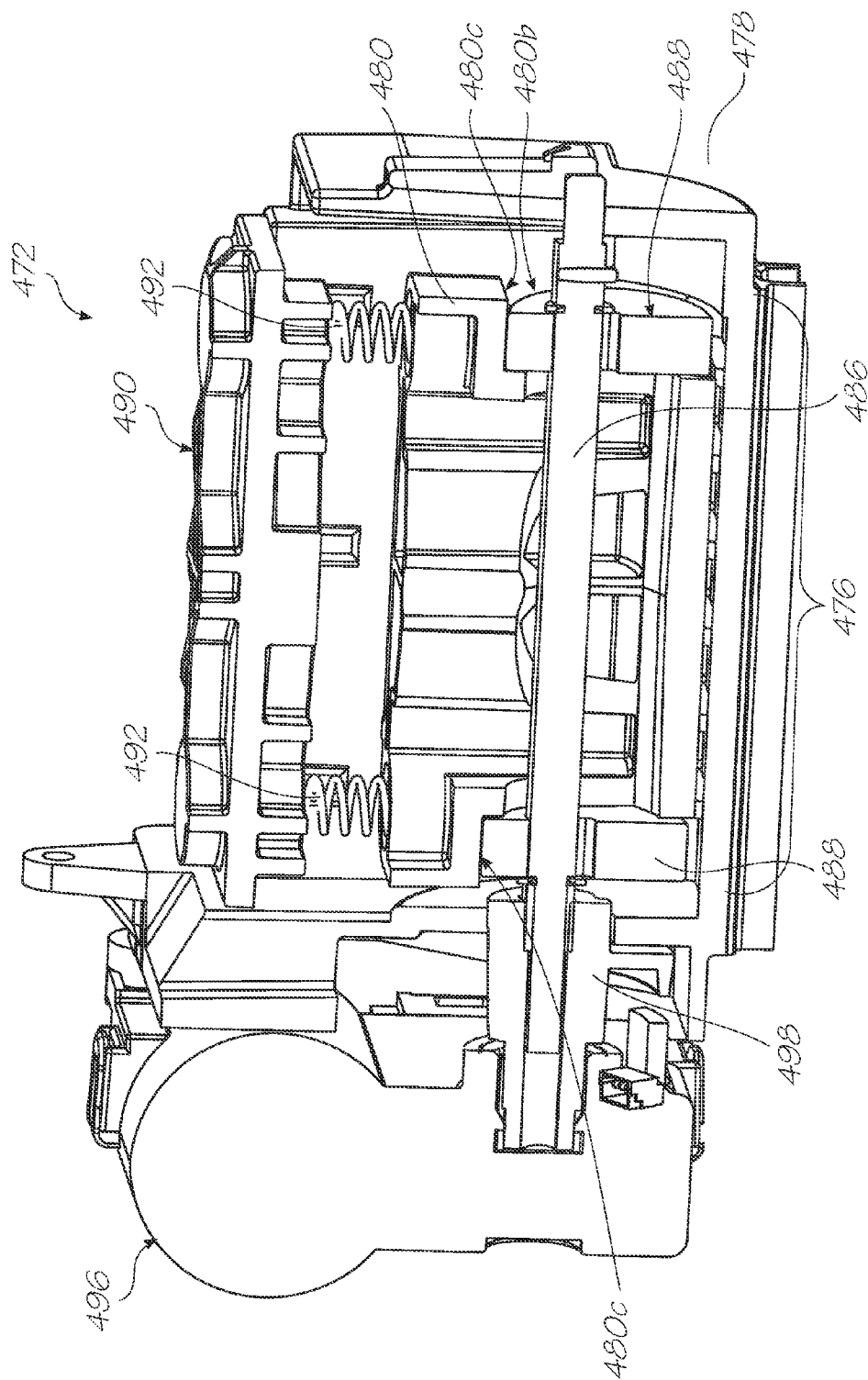
FIG. 41B
