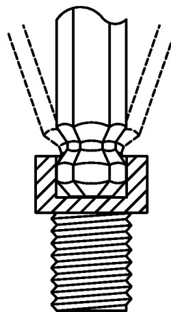
FIG. 8D
