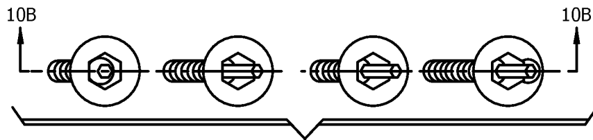
FIG. 10A
