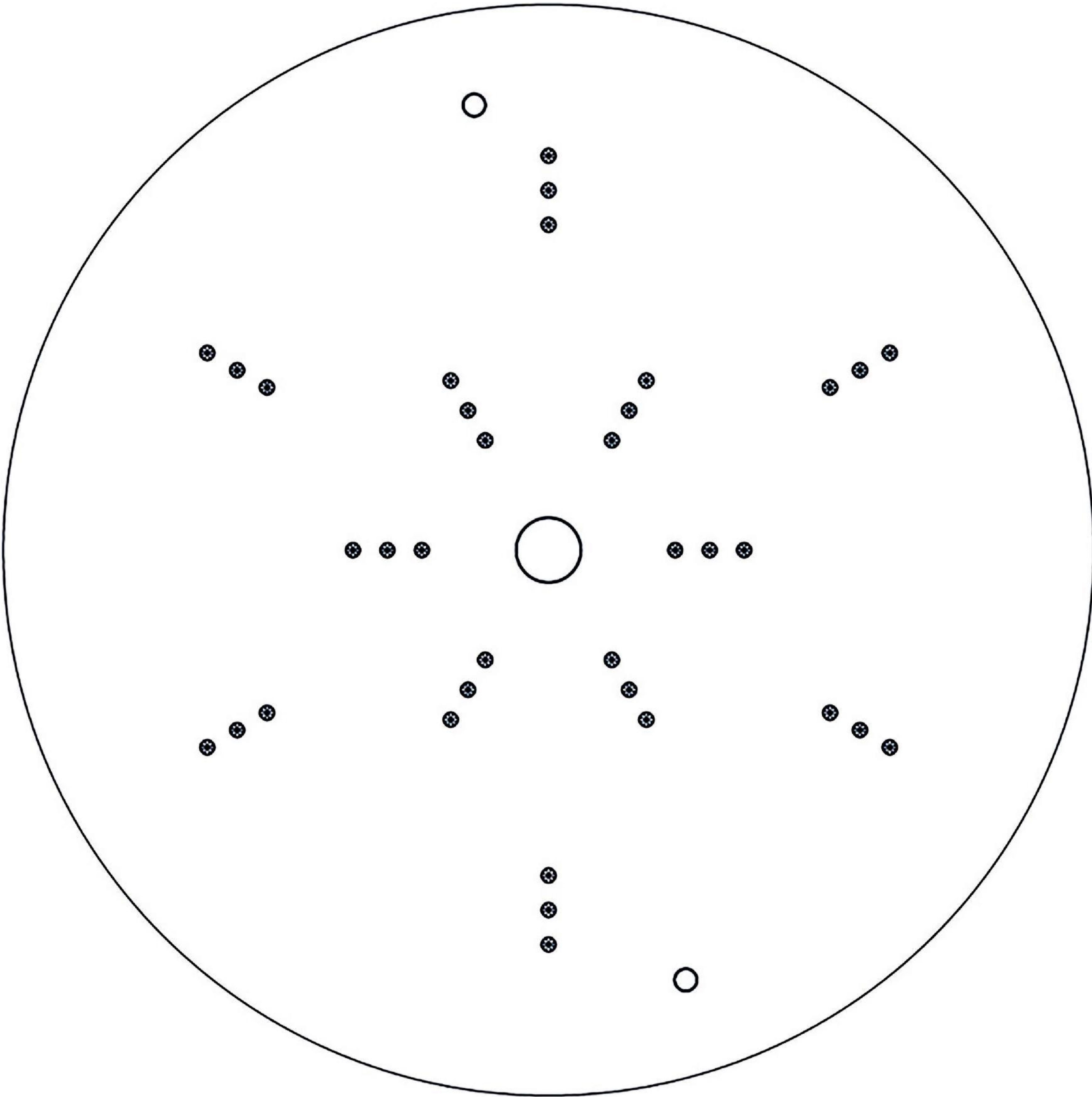
【後視圖】
