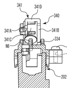
(B) T-T断面図
