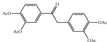
bis(3,4-diacetoxy)desoxybenzoin
