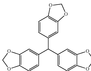
Tris-(3,4-methylenedioxyphenyl)methane
