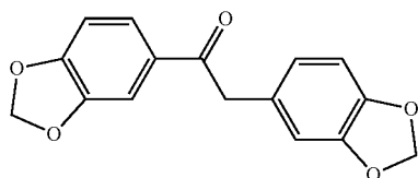
bis(3,4-methylenedioxy)desoxybenzoin
