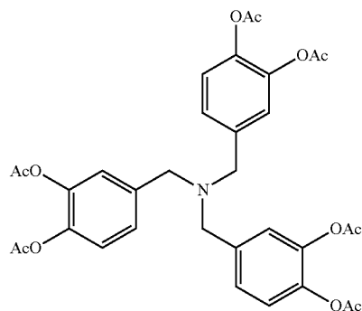
tris-(3,4-diacetoxybenzyl)-amine
