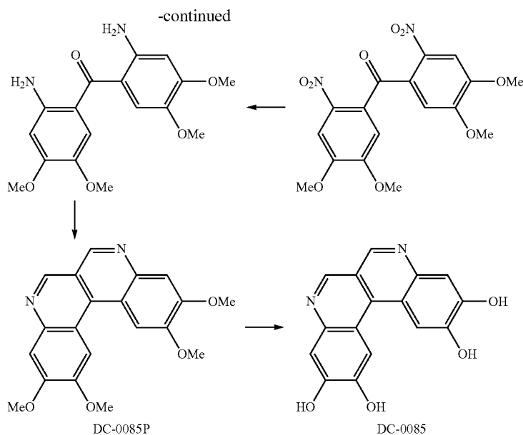
2,3,10,11-Tetramethoxydibenzo[c,f][2,7]naphthyridine (DC-0085P)
