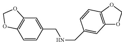
bis-(3,4-methylenedioxybenzyl)-amine
