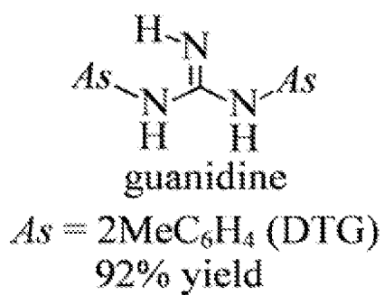
DTG
