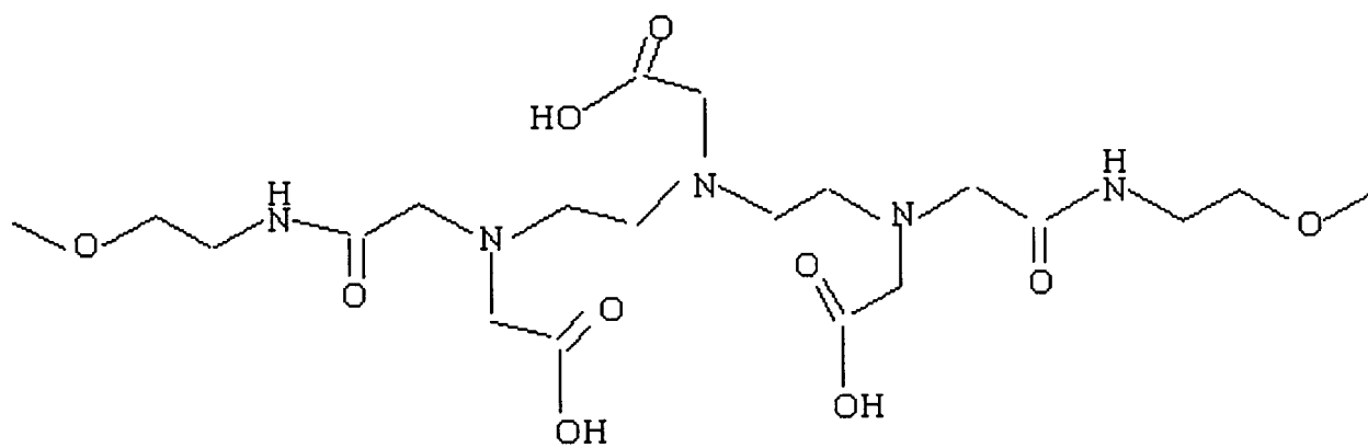
DTPA-BMEA
