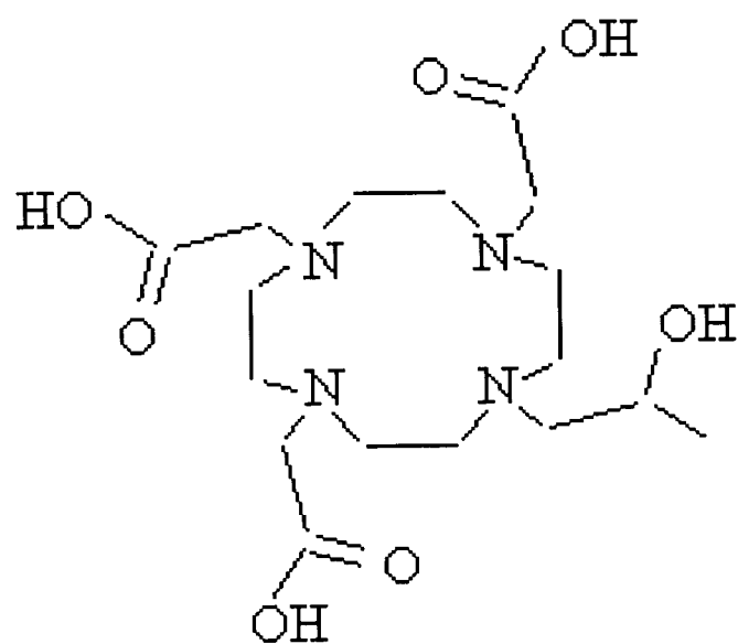
DOTA
