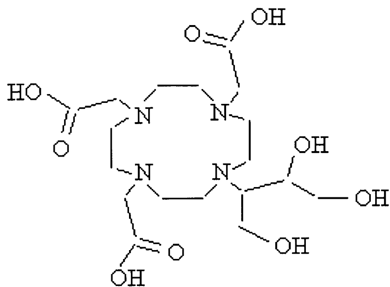
DO3A-butrol
