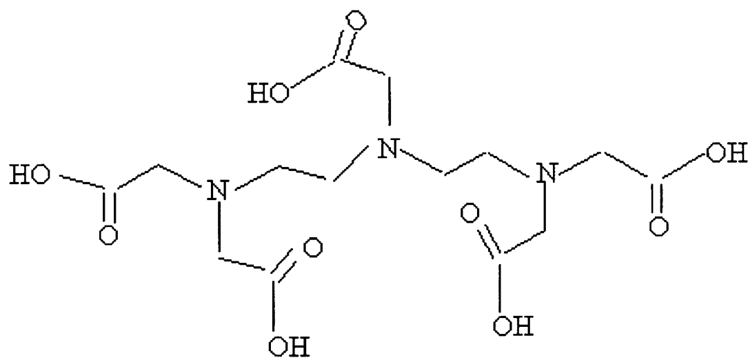
DTPA
