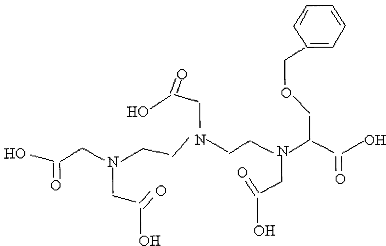
DTPA-BMEA
