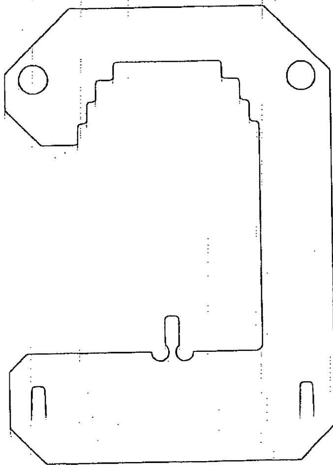
Pladeophæng til væksthussarmaturer fig. 1
