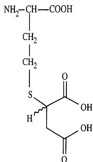
S -2-( 2R , 2S -SUCCINYL)-DL-HOMOCYSTEINE
