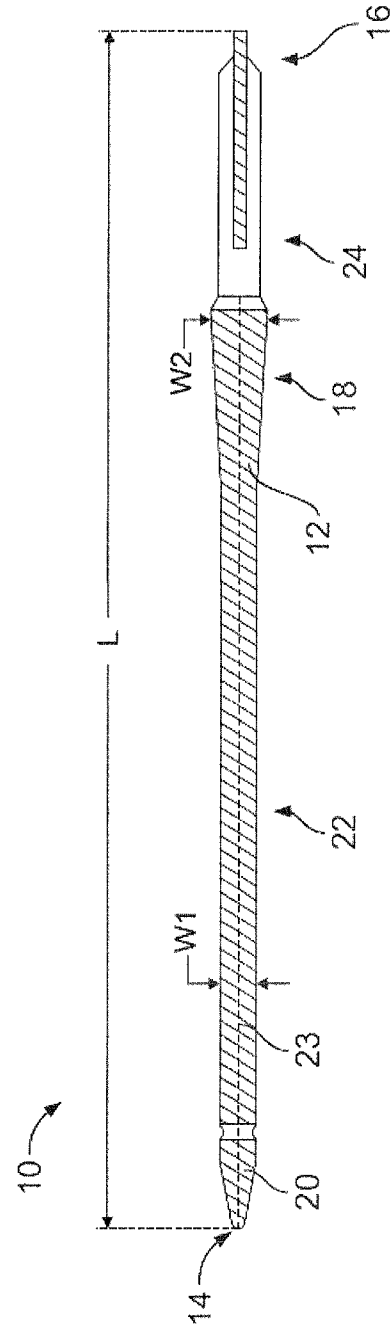
FIG. 2B (Along A-A)
