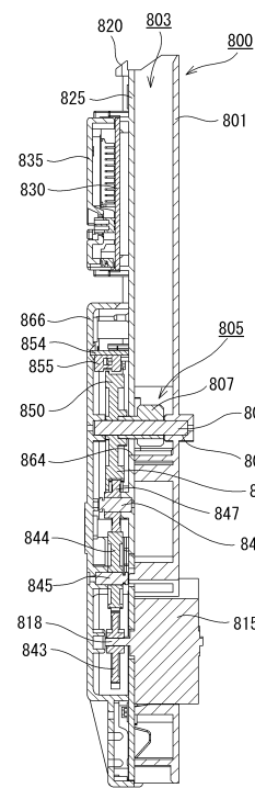
A-A断面図
