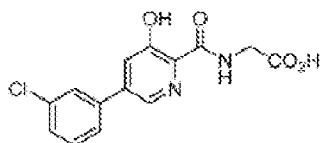
Forbindelse 1
