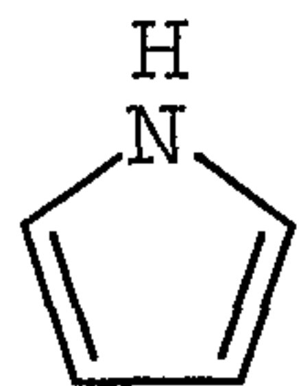
pyrrolyl
