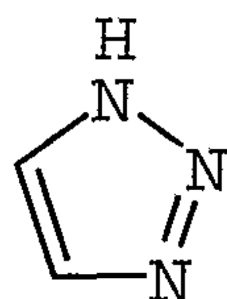
1,2,3-triazolyl
