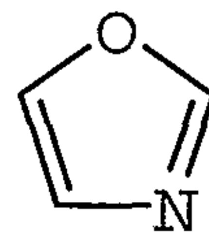
oxazolyl
