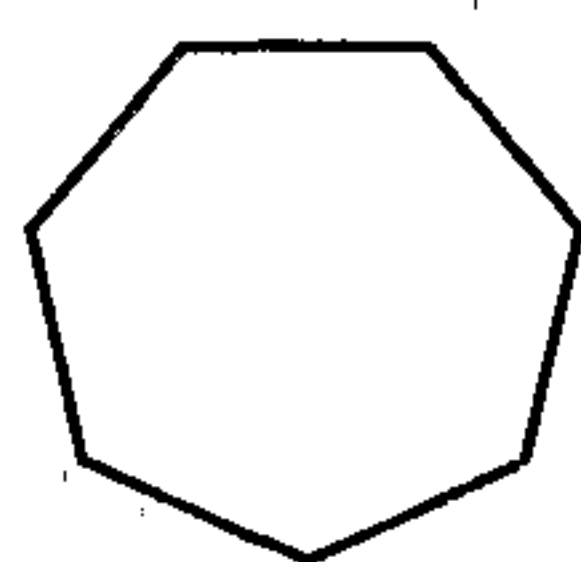
cycloheptyl
