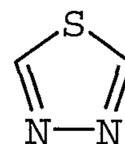
1,3,4-thiadiazolyl
