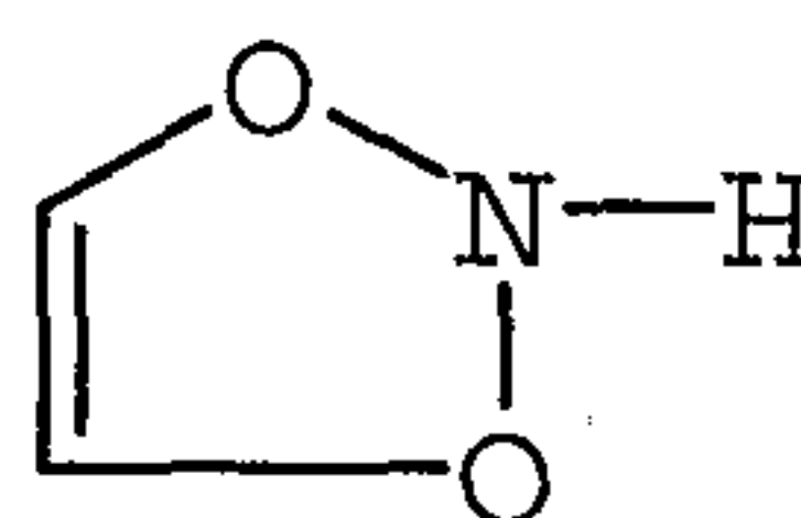
1,3,2-dioxazolyl
