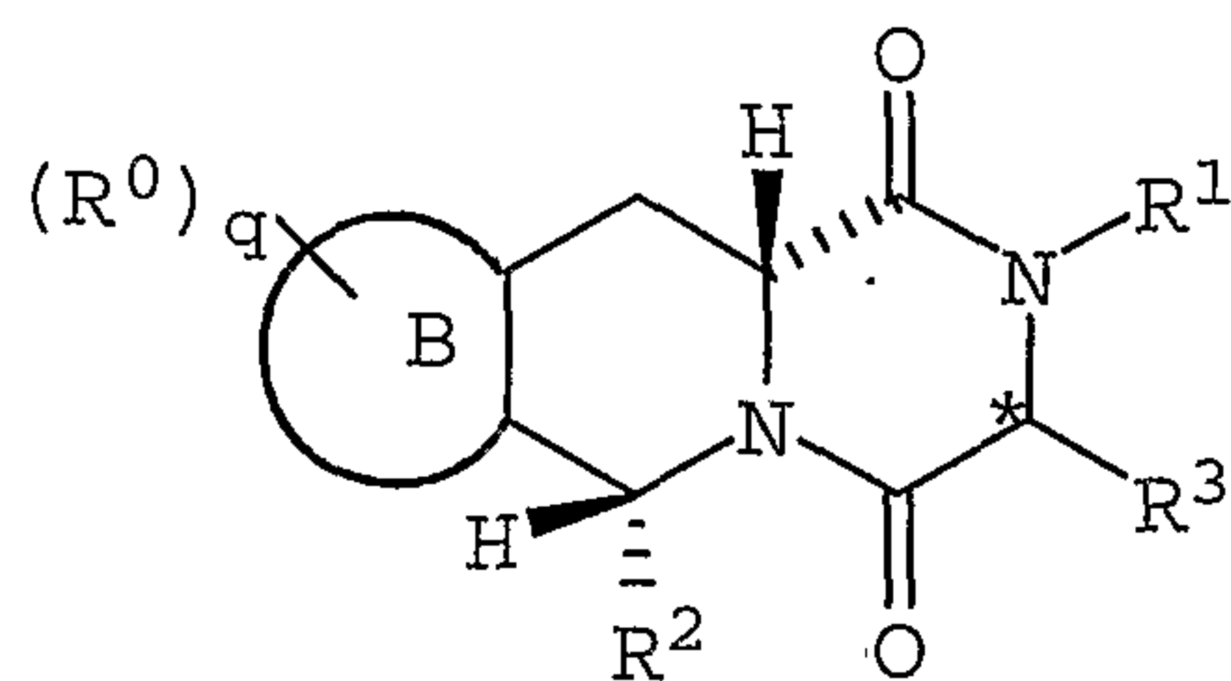
(II)
