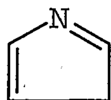
3H-pyrrolyl
