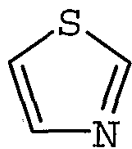
thiazolyl
