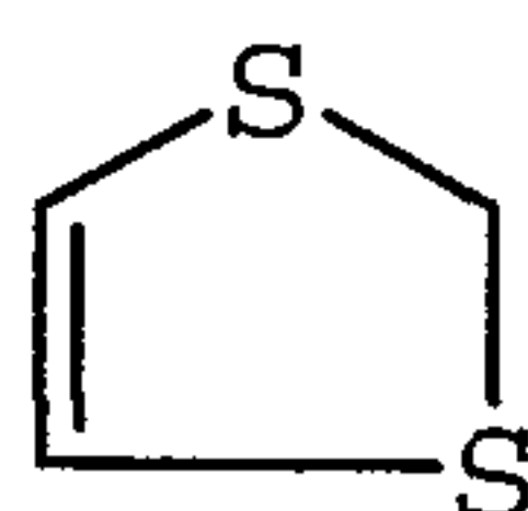
1,3-dithiolyl
