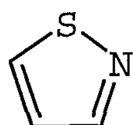
isothiazolyl
