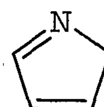
2H-pyrrolyl
