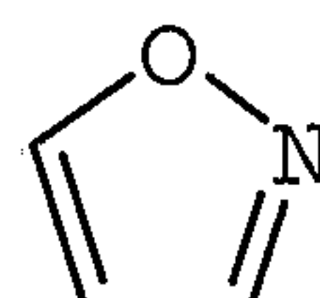
isoxazolyl
