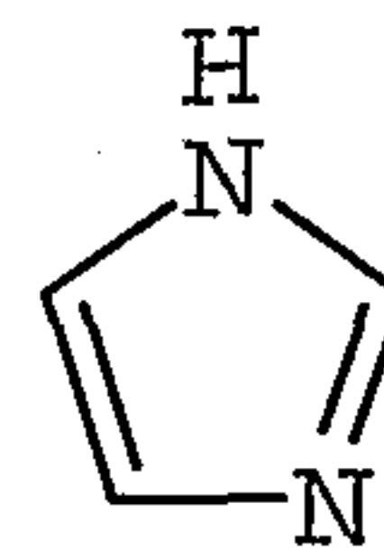
imidazolyl
