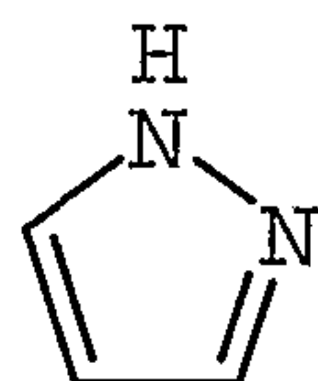
pyrazolyl
