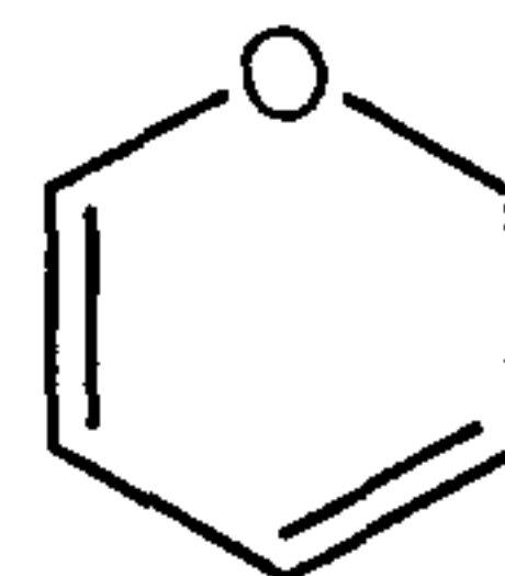
2H-pyranyl
