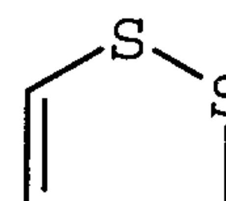
1,2-dithiolyl
