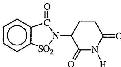
supidimide.
