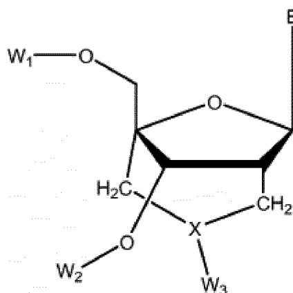
Formule I
