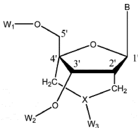
Formule I
