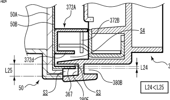
【図13-51】 開閉扉枠底部品 (特定内部進入部品と被進入部品/ドア枠所定部品と内枠所定部品)
