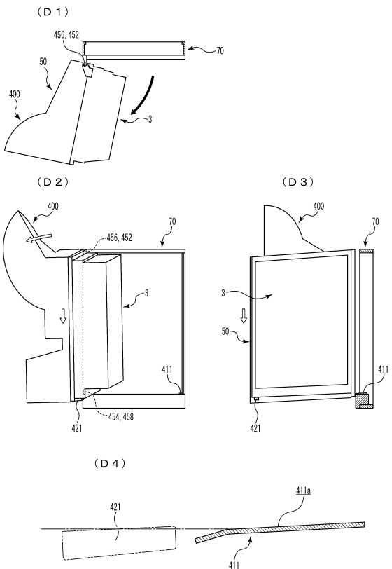
【図13-48】 遊技機用枠+開閉扉枠 [第4開状態 (開放角度: 約90度)]
