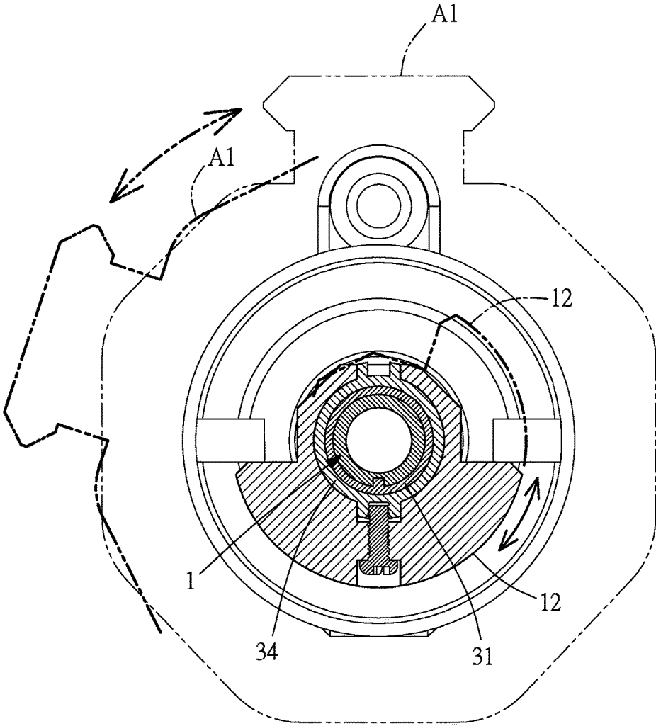
B-B' FIG. 7
