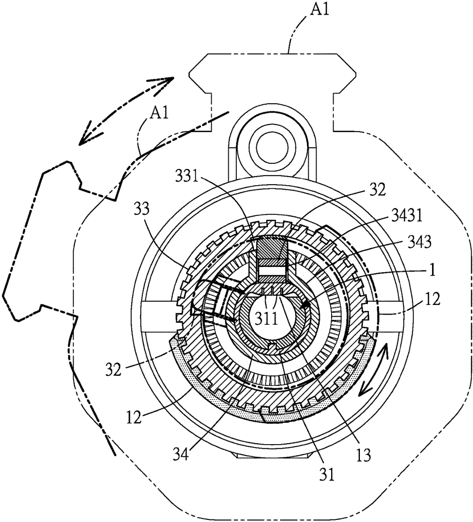
A-A' FIG. 6
