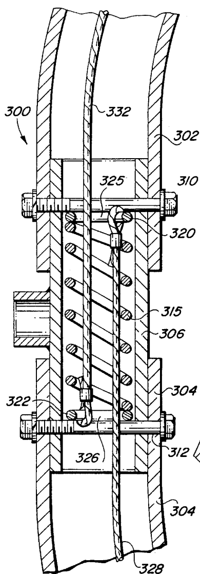
FIG. 19
