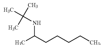
N-tert-butylheptan-2-amine:
