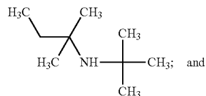
N-tert-butylheptan-2-amine:
