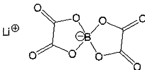
[Chem. 85]
