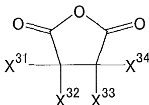
[Chem. 55]
