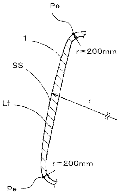
Cross-section E1
