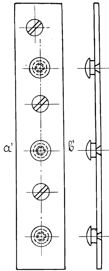
przekrój a'.b'.
