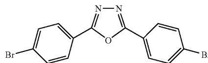
2,5-Bis-(4-bromo-phenyl)-[1,3,4]oxadiazole
