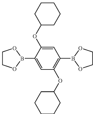
2,5-Bis-(4-bromo-phenyl)-[1,3,4]oxadiazole
