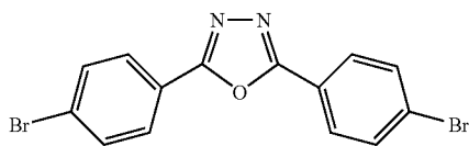
2,5-Bis-(4-bromo-phenyl)-[1,3,4]oxadiazole
